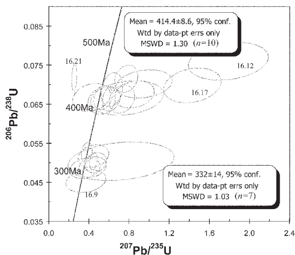
图 4 克拉玛依蛇绿岩带中蚀变辉长岩样品 05KBK-16 锆
