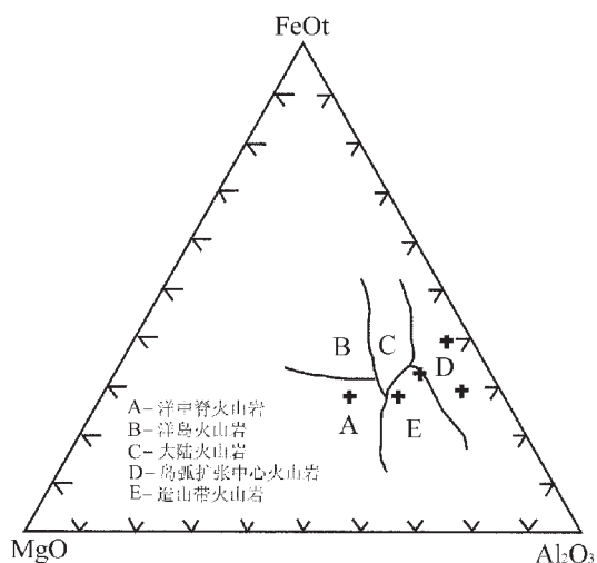
图 3 克拉玛依蛇绿岩带中玄武岩的
