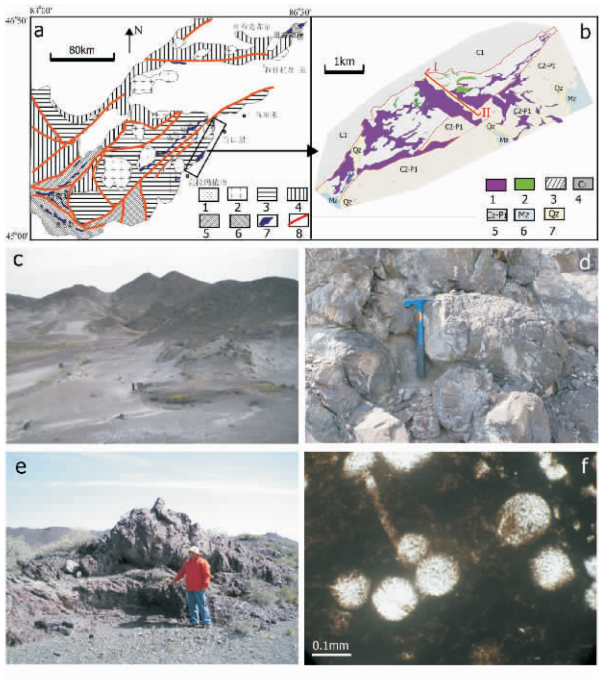
图 1 a—西准噶尔地区蛇绿岩分布图(方框示本次研究区范围):1—中—新生代;2—晚古生代花岗岩;3—石炭系;4—泥盆系;5—志留系;6—奥陶系;7—蛇绿岩;8—断层;b—克拉玛依蛇绿岩体地质图(I—II 示实测剖面位置):1—超镁铁岩;2—镁铁岩;3—增生杂岩;4—下石炭统太勒古拉组;5—上石炭—下二叠统;6—中生界;7—第四系;c—克拉玛依蛇绿岩的野外露头;d—枕状玄武岩;e—硅质岩;f—和在硅质岩中发现的放射虫
