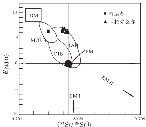
图 5 Sr—Nd 二元相关图(据 Zindler [25] )
