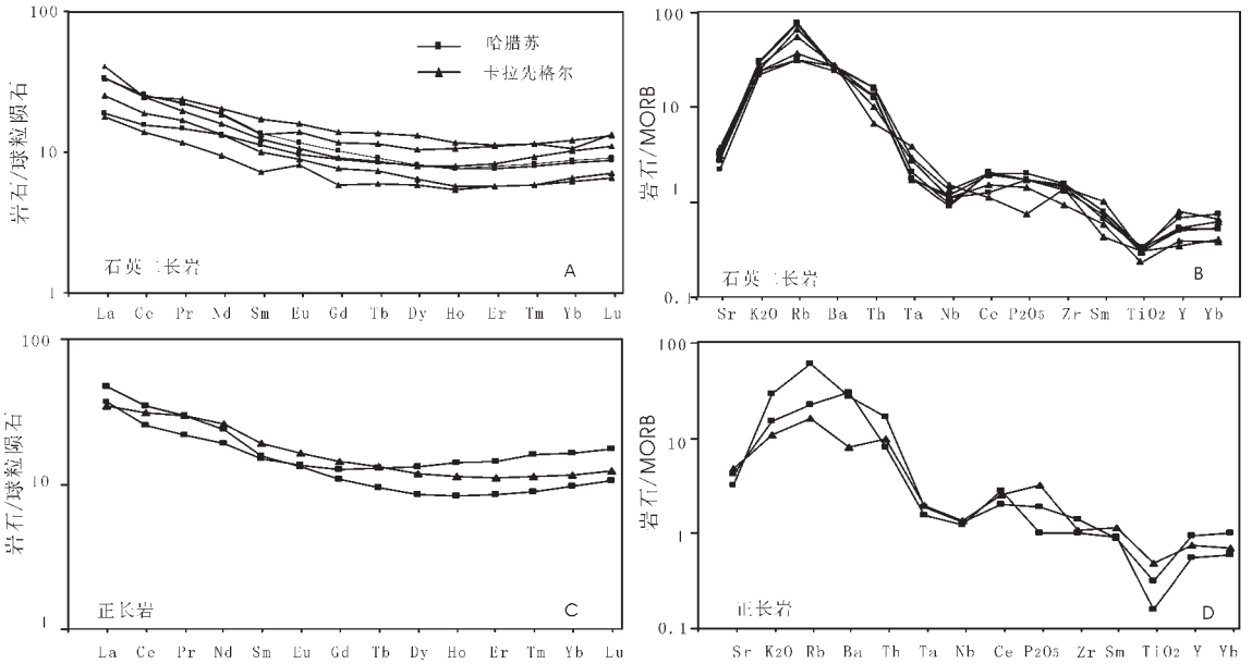
图3 含矿斑岩稀土配分图及微量元素蛛网图 [11]
