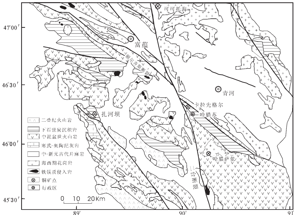
图 1 阿尔泰南缘卡拉先格尔区域及矿产分布图(据参考文献[2]修改)
