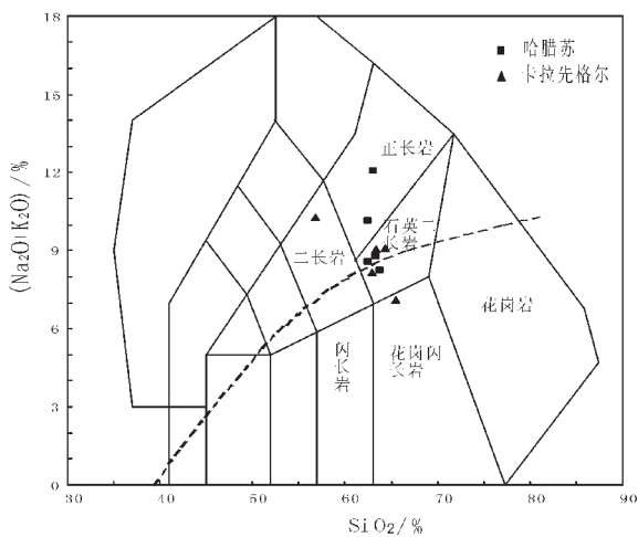
图 2 矿区火成岩 TAS 图 (碱性亚碱性分界线据 Irvine [9] )
