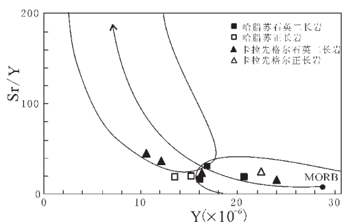
图 6 Sr/Y—Y 二元相关图解(据 Defant [9] )
