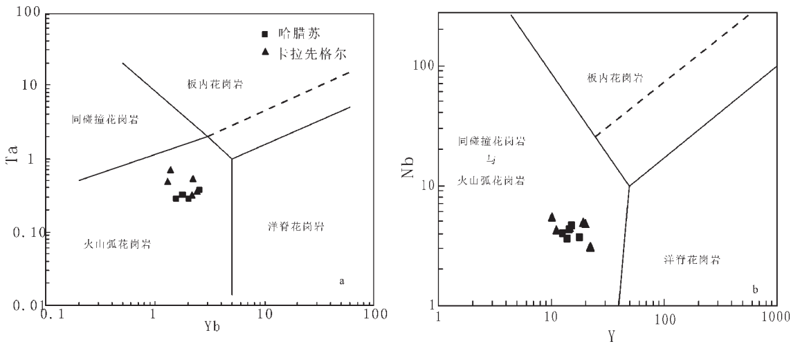
图4 花岗岩类 Ta—Yb(a)和 Nb—Y(b)构造判别图 [23]
