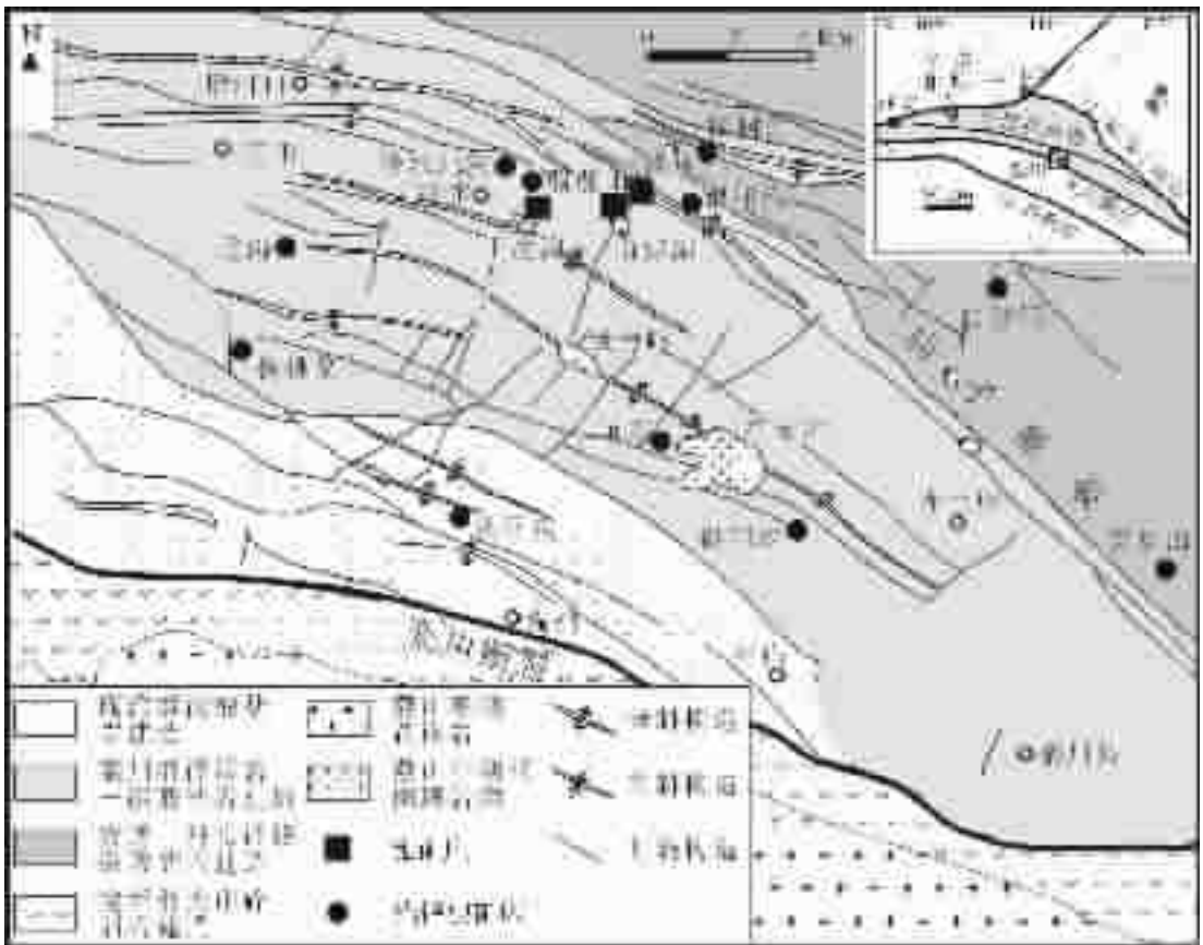
图 7 河南冷水北沟铅锌银矿床区域地质简图 [36]
