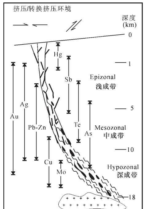
图3 矿床尺度的造山型矿床成矿模式——地壳连续模式 Fig.3 Crustal continuum model for orogenic-type deposits: deposit-scale
