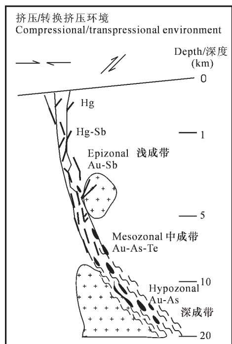
图 1 造山型金矿的地壳连续模式 [9]
