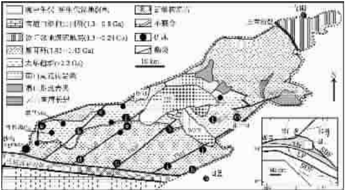
图 11 熊耳地体地质和矿床分布图
