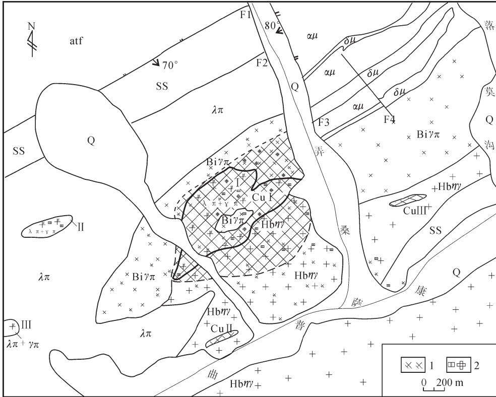
图 4 西藏朱诺斑岩铜矿地质简图
