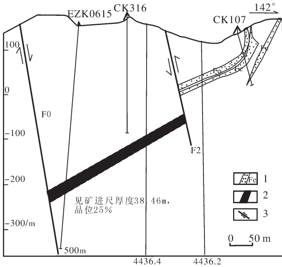
图12 河北迁安铁矿二马铁矿床N200勘探线剖面图 ① 1—已知矿体;2—新发现矿体;CK—以往施工钻孔; ZK—本次施工钻孔;5—断层
