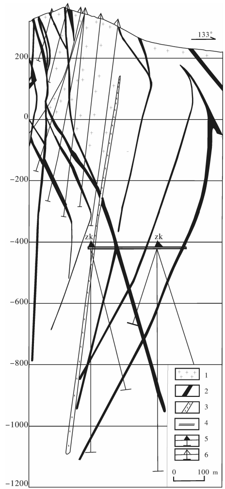
图8 山东玲珑金矿175号群脉71线剖面图 ①
