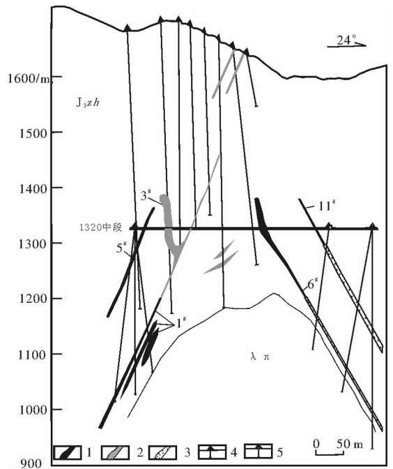
图5 山西支家地6号勘查线剖面图②
