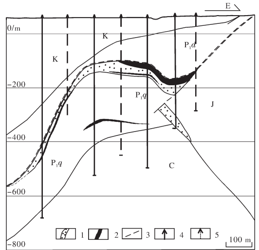
图3 湖南康家湾铅锌矿147线剖面图 ③
