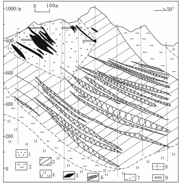
图20 福建紫金山铜金矿3线蚀变岩分带地质剖面图 1—硅质交代岩带;2—石英迪开石蚀变岩带;3—石英明矾石蚀变岩带;4—石英绢云母蚀变岩带;5—金矿体;6—铜矿体; 7—蚀变岩界线;8—钻孔;9—穿脉坑道
