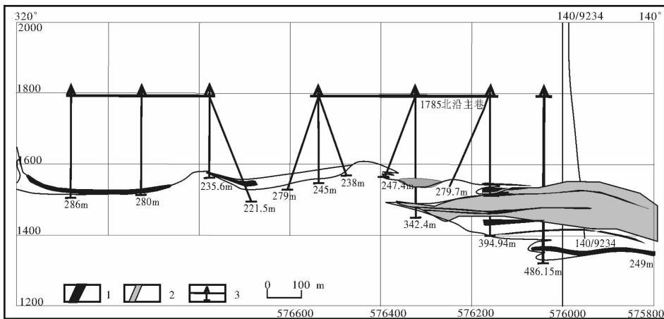
图7 云南个旧老厂D10线地质剖面图②
