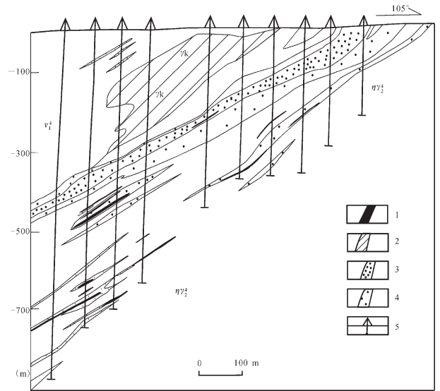
图17 山东寺庄矿区280勘探线地质剖面图 ①
