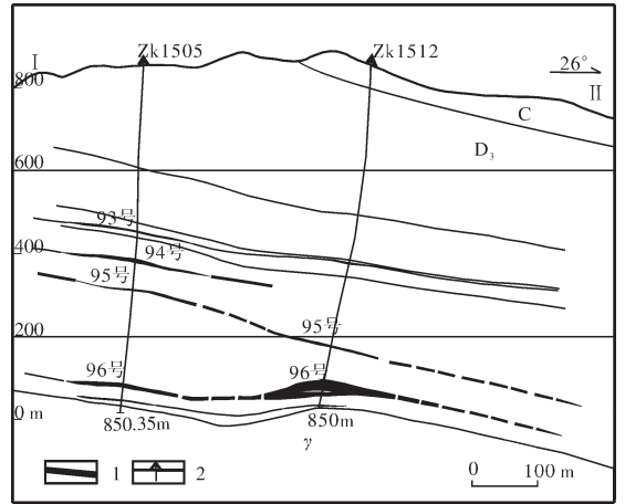
图2 广西南丹铜坑锡矿1号线剖面图 ②
