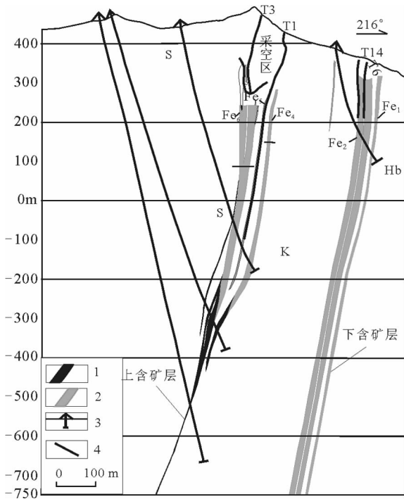
图1 辽宁弓长岭铁矿床二矿区20线剖面图 ①
