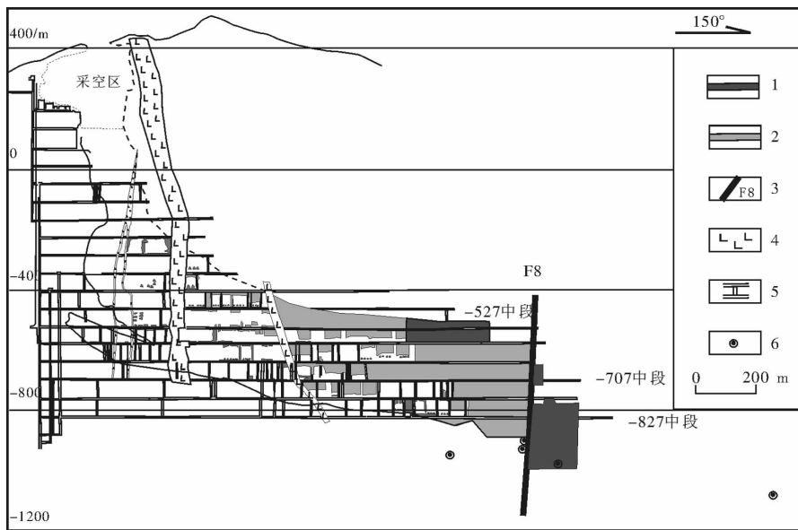
图11 辽宁红透山铜锌矿床3号矿体垂直纵投影图①
