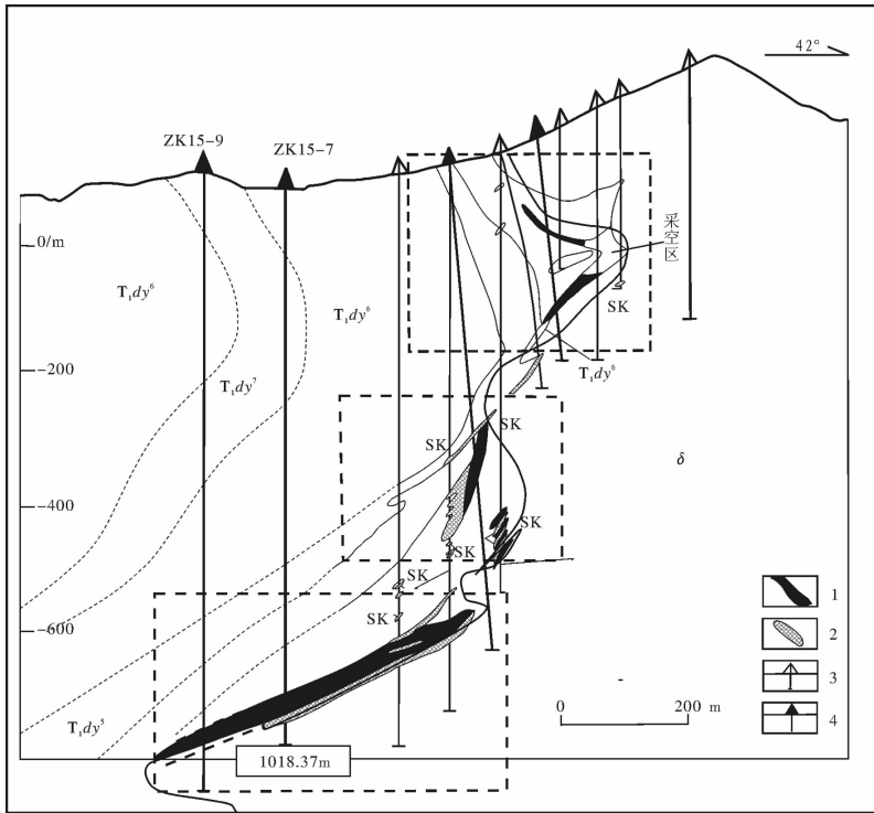
图6 湖北大冶铁矿床15勘探线设计剖面图①
