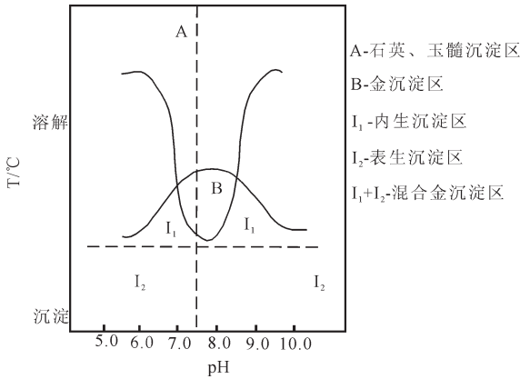
图13 金沉淀温度与酸碱度关系(据陈光远,1986)
