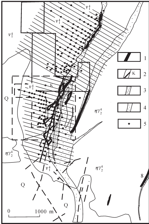
图16 山东焦家金矿带南段综合地质图 ①
