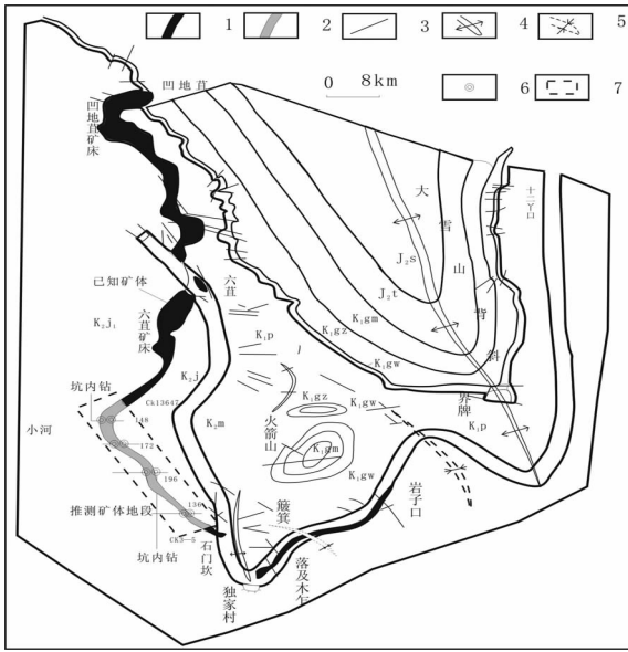
图4 云南大姚六直铜矿地质略图①
