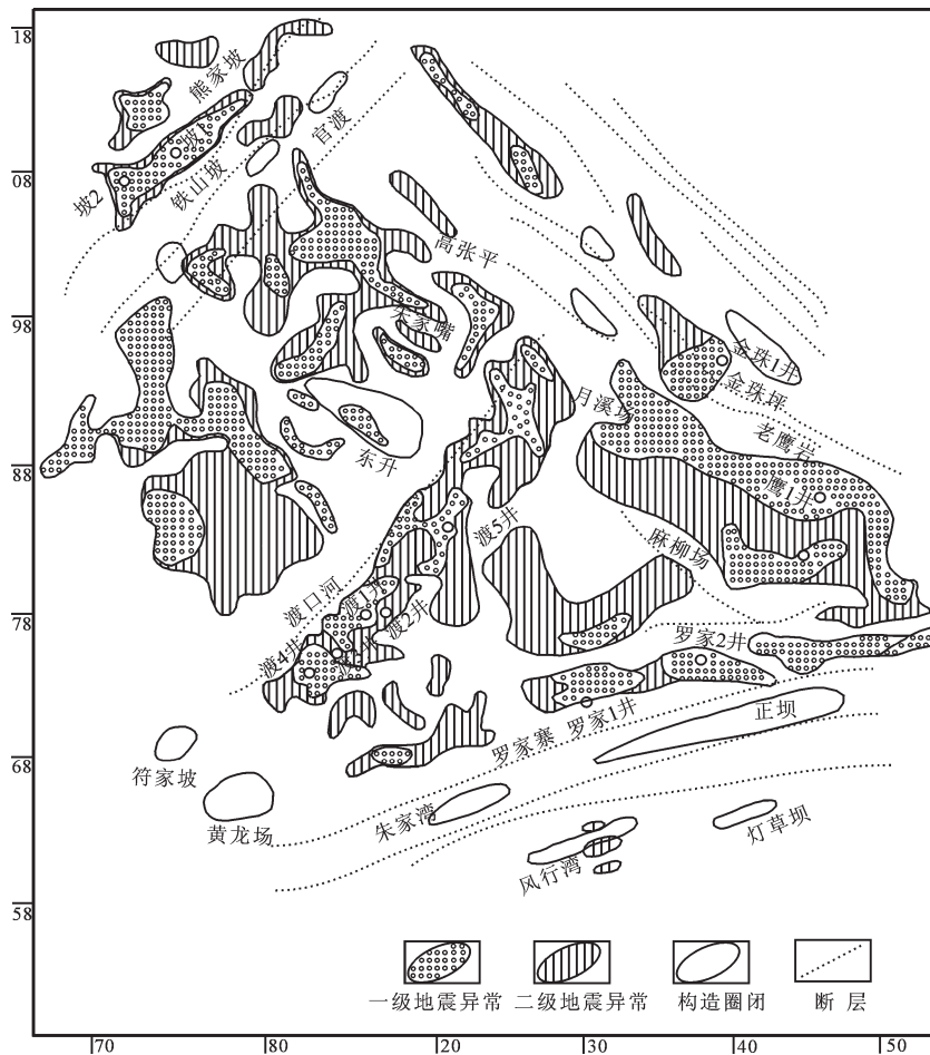
图 13 飞仙关组储层地震横向预测图
