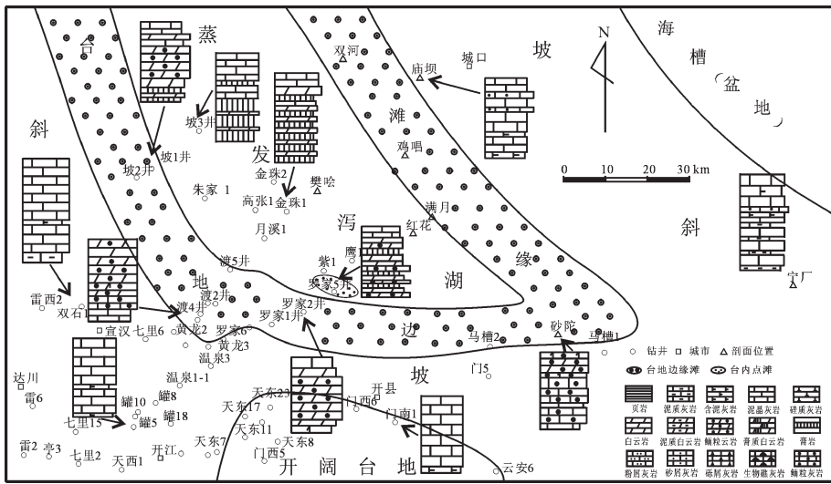
图6 川东北地区早三叠世飞二段时期孤立碳酸盐岩台地沉积相平面展布图
