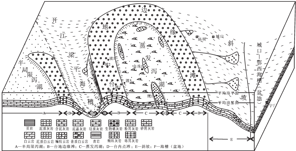
图 4 川东北地区飞一—飞三段时期孤立碳酸盐台地沉积立体模式图
