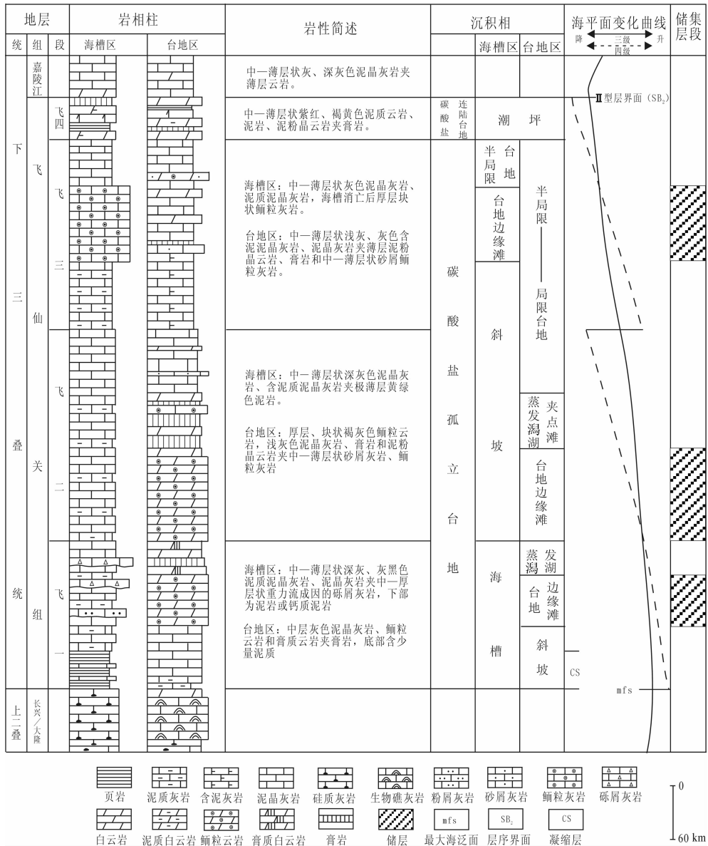
图3 川东北地区下三叠统飞仙关组地层、海平面变化及特征简图
