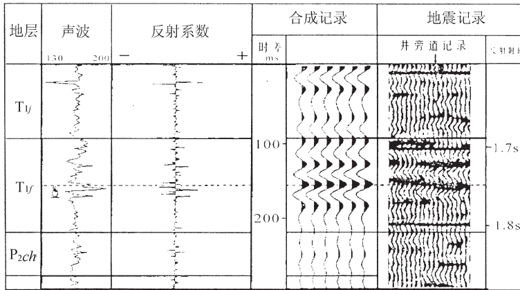
图 12 渡 1 井飞仙关组鲕滩储层声波地震合成记录
