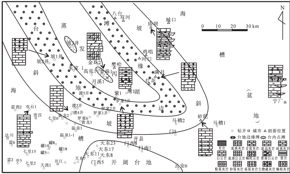
图5 川东北地区早三叠世飞一段时期孤立碳酸盐岩台地沉积相平面展布图
