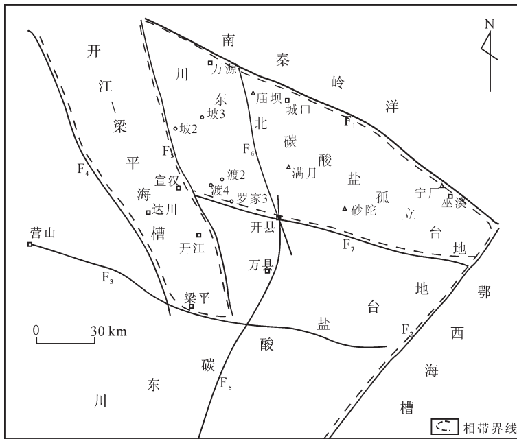
图 2 基底断裂及沉积相分布图
