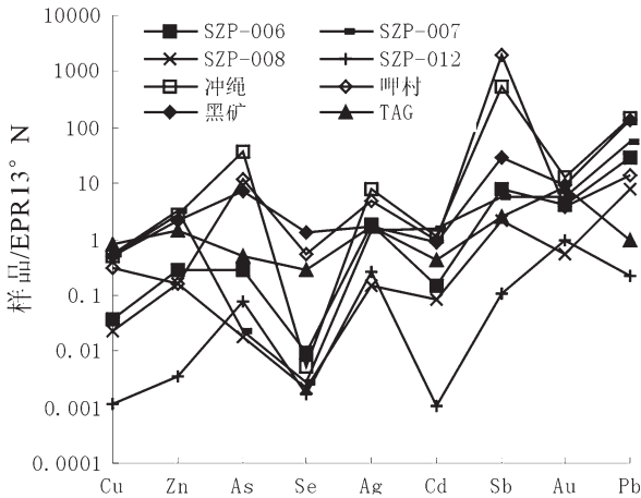
图5 上庄坪及典型 VMS 型矿床(岩)石微量元素配分形式(EPR13°N 标准化 [19] )
