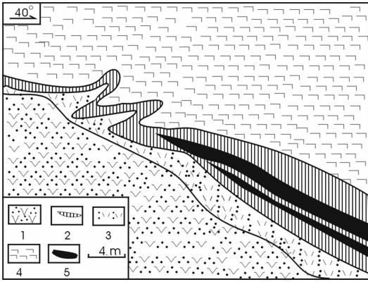
图 2 嵩县上庄坪铅锌银矿床地质剖面图 1—石英角斑岩;2—矿化重晶石岩;3—凝灰岩; 4—细碧岩;5—硅质岩
