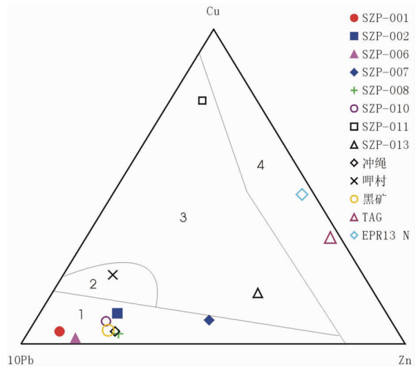
图6 上庄坪矿床 Cu-Pb-Zn 构造环境判别图解(底图数据据参考文献[17])
