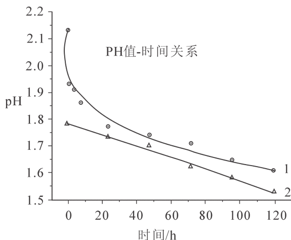
图 5 细菌处理过程中 pH 值-时间关系
