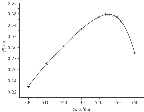
图 2 Au-TMK 体系吸光度曲线 ( 8 \times 10^{-6}\text{Au} , 2cm 比色皿)
