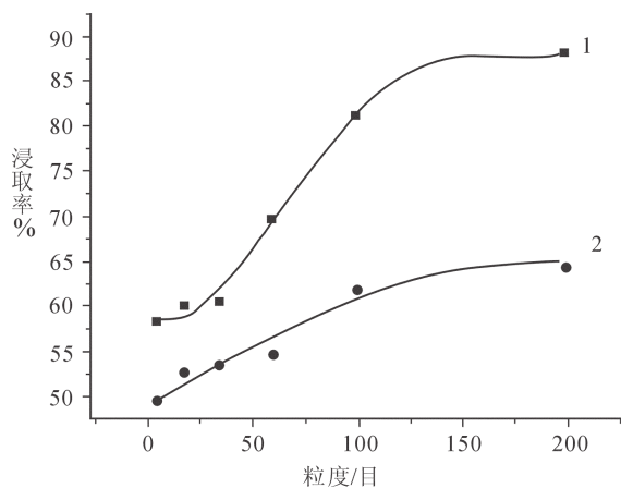
图 4 浸取率与矿石粒度的关系
