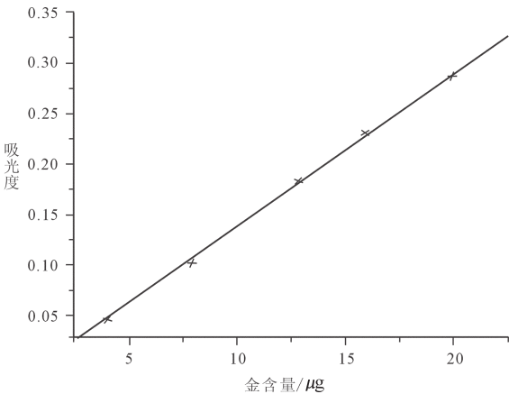
图 3 Au 含量工作曲线 (波长 545 nm, 2 cm 比色皿)
