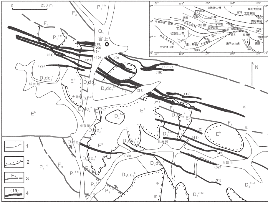
图1 寨上金矿床矿区地质略图(武警黄金部队第五支队提供,2006)
