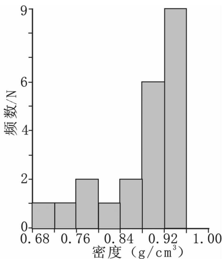
图 4 乌拉嘎金矿成矿流体密度直方图
