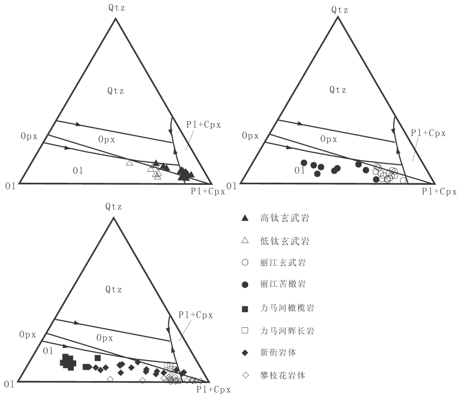
图 5 Ol-Qtz-Pl+Cpx 相图 [38]
