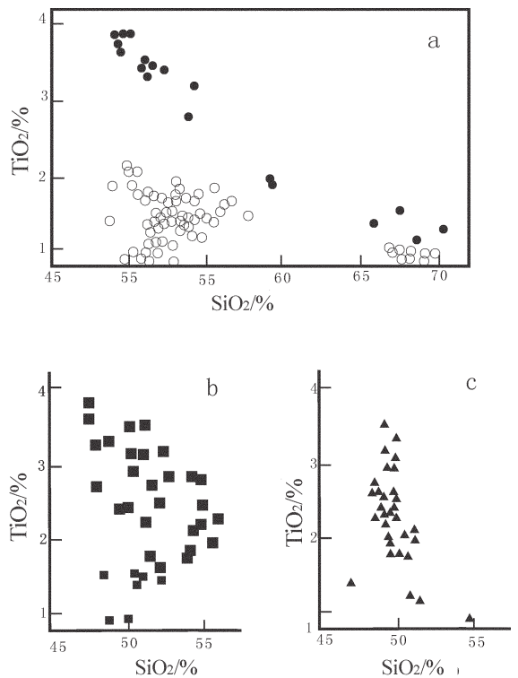
图 1 SiO 2 -TiO 2 图解。
