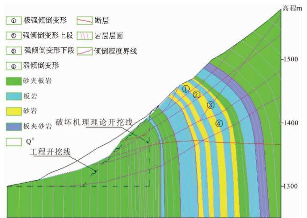
图 3 右坝肩边坡工程地质剖面图
