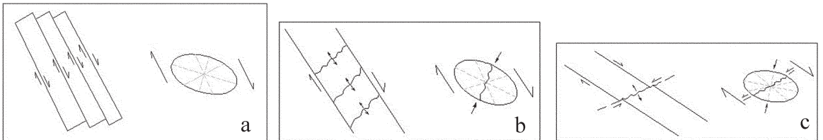
图 11 不同倾倒变形程度岩体的破裂形式及力学机制 a—弱倾倒层内剪切错动;b—强倾倒层间张拉变形;c—强倾倒切层张性剪切破裂
