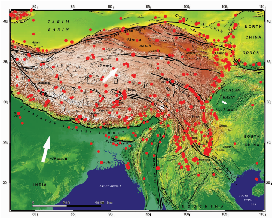
图 2 青藏高原地震震中分布与动力学模型图 [48-49]
