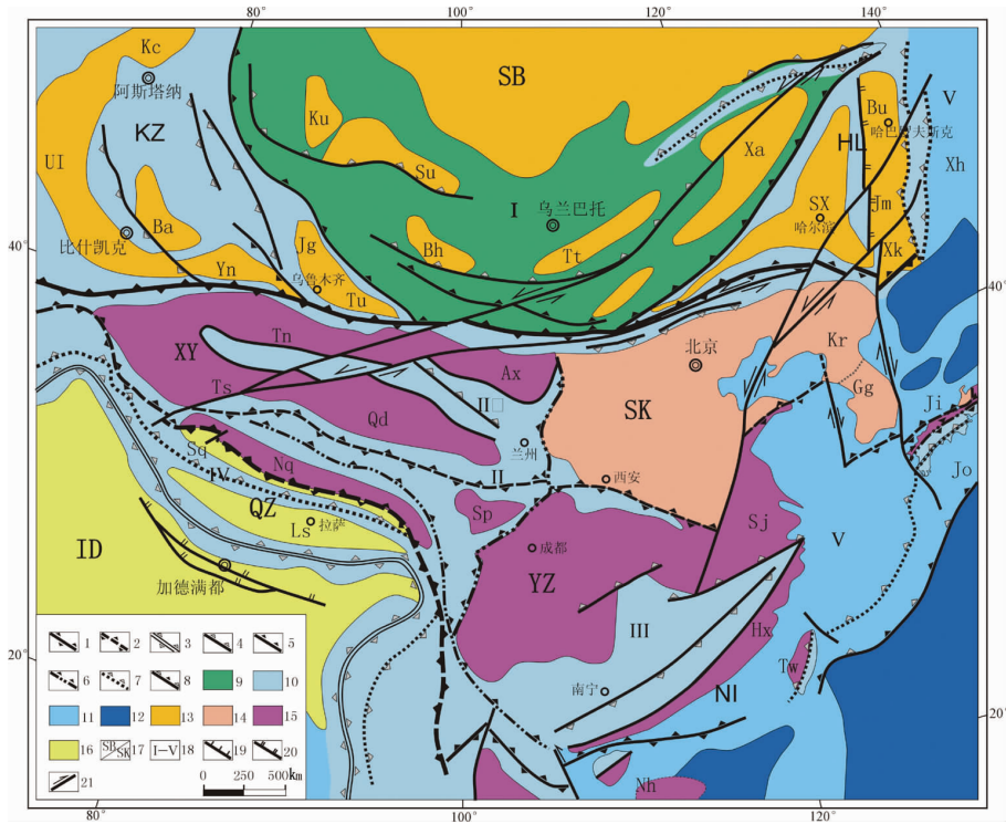
图 1 晚中生代—新生代中国及邻区大地构造略图(据王鸿桢, 1990 [20] 改编)
