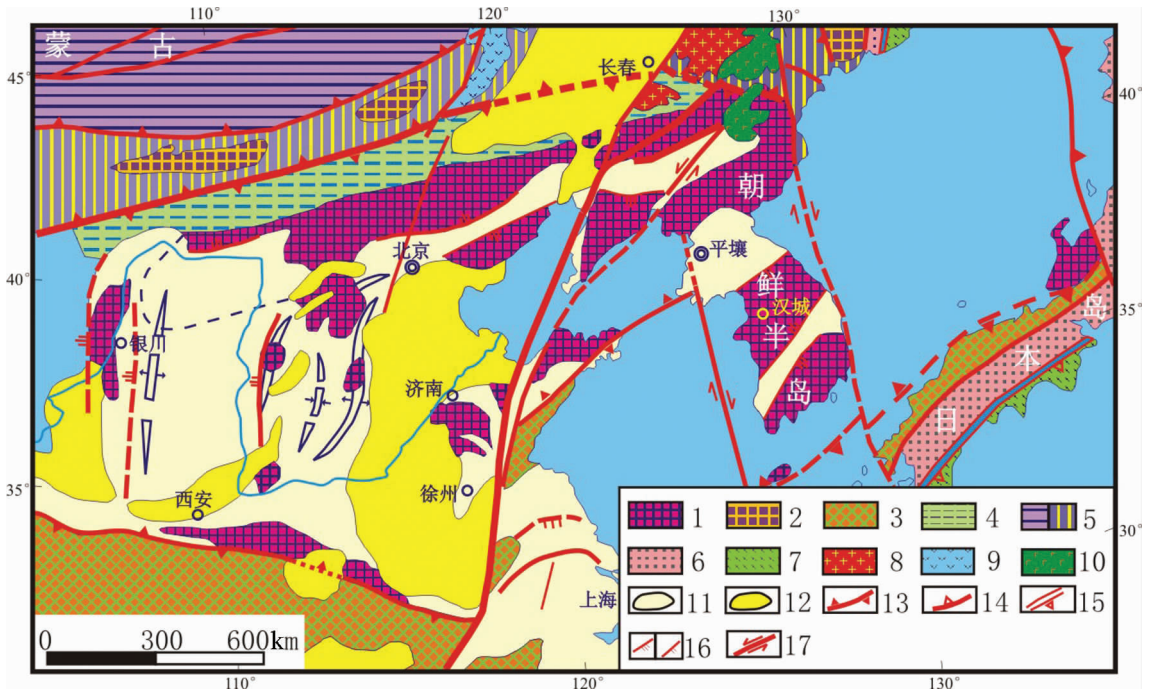
图 3 中朝板块与邻区大地构造略图
