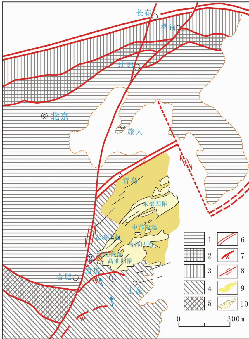
图4 苏北—南黄海背景构造略图
