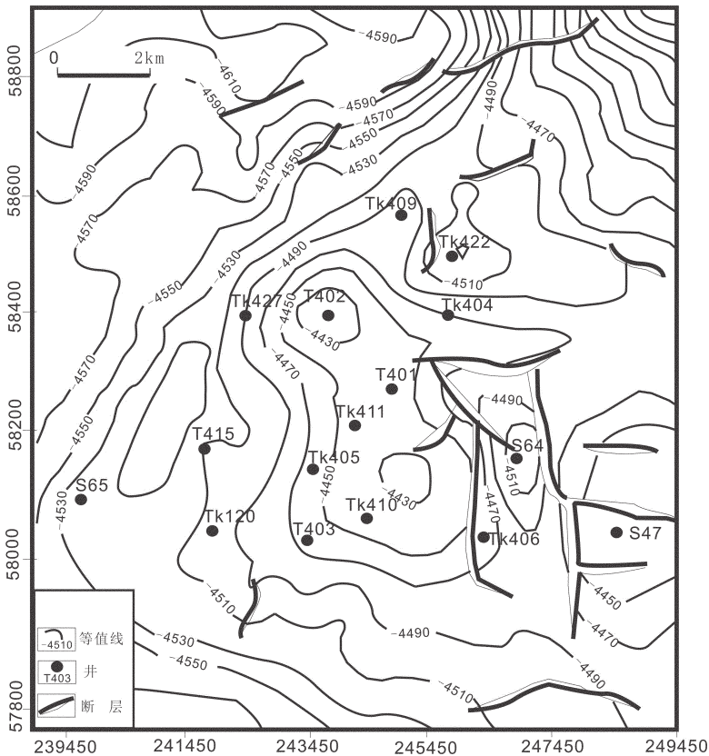
图2 塔河四区奥陶系构造图
