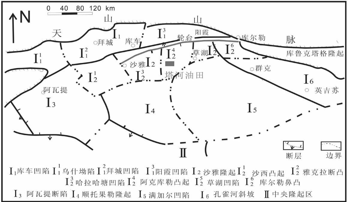
图1 新疆塔里木盆地塔河油田奥陶系油藏构造位置
