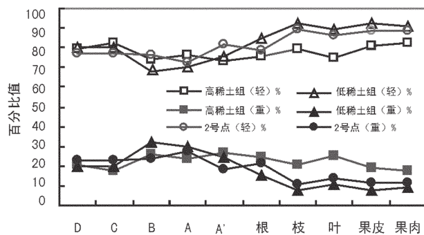
图 4 岩土脐橙系统中轻、重稀土百分比值分馏趋势图
