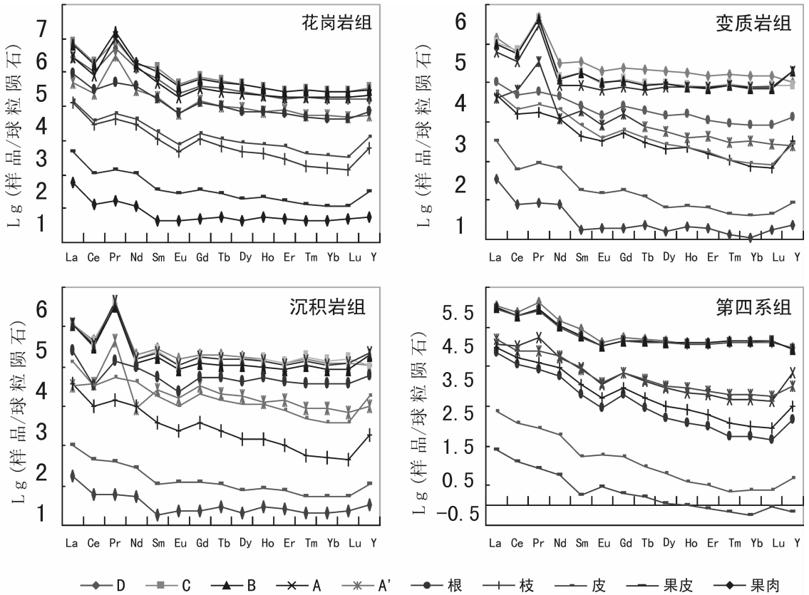
图 1 岩-土-脐橙系统稀土元素分配曲线
