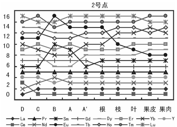
图 5 2 号点岩土脐橙系统中稀土元素百分比值次序图
