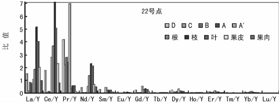
图 3 演化、迁移过程中稀土元素分馏分异趋势图
