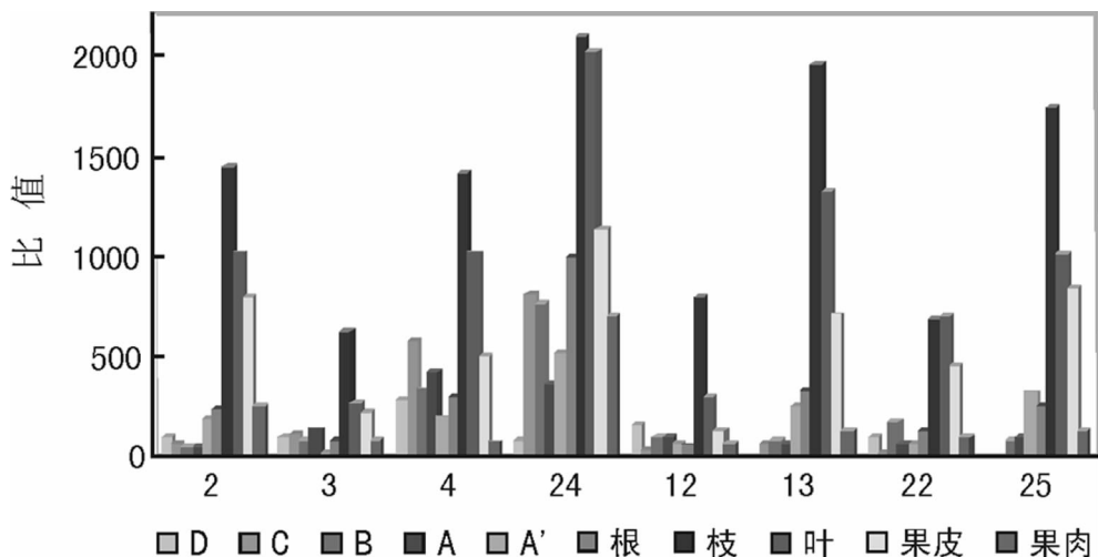
图 2 岩-土-脐橙系统的 La/Lu 值变化趋向图
