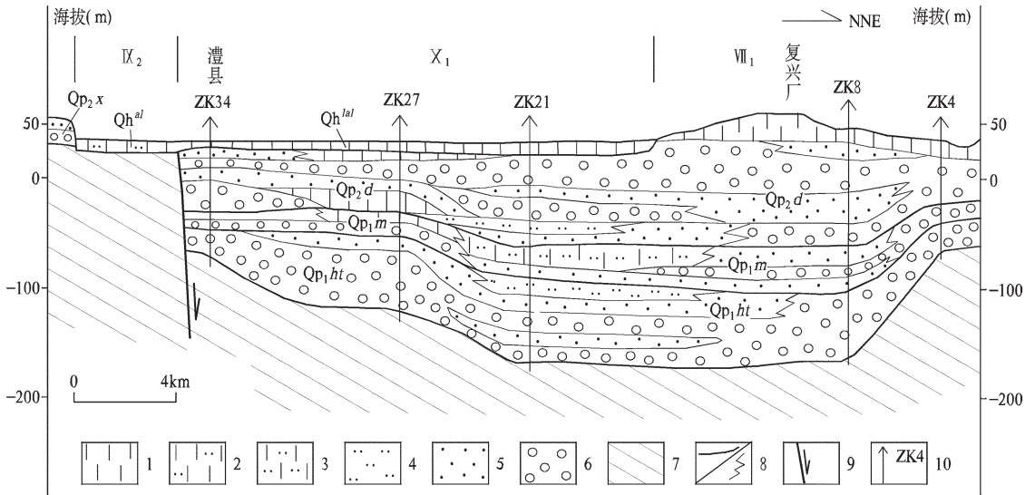
图 9 复兴厂—澧县第四纪地质地貌剖面(剖面位置见图 2)
