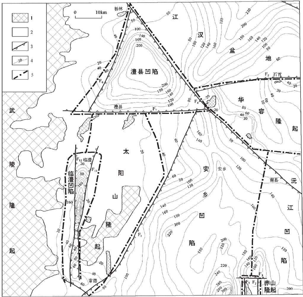
图 1 研究区第四纪构造格局
