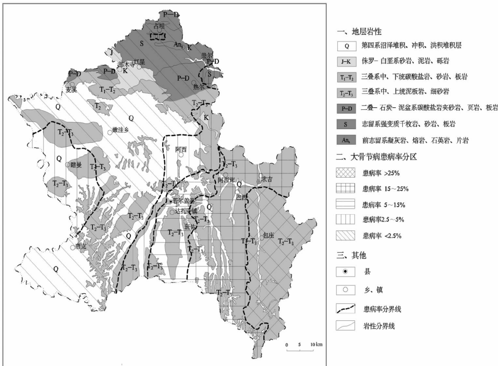
图 3 若尔盖县岩性分布与大骨节病患病率分布对照图
