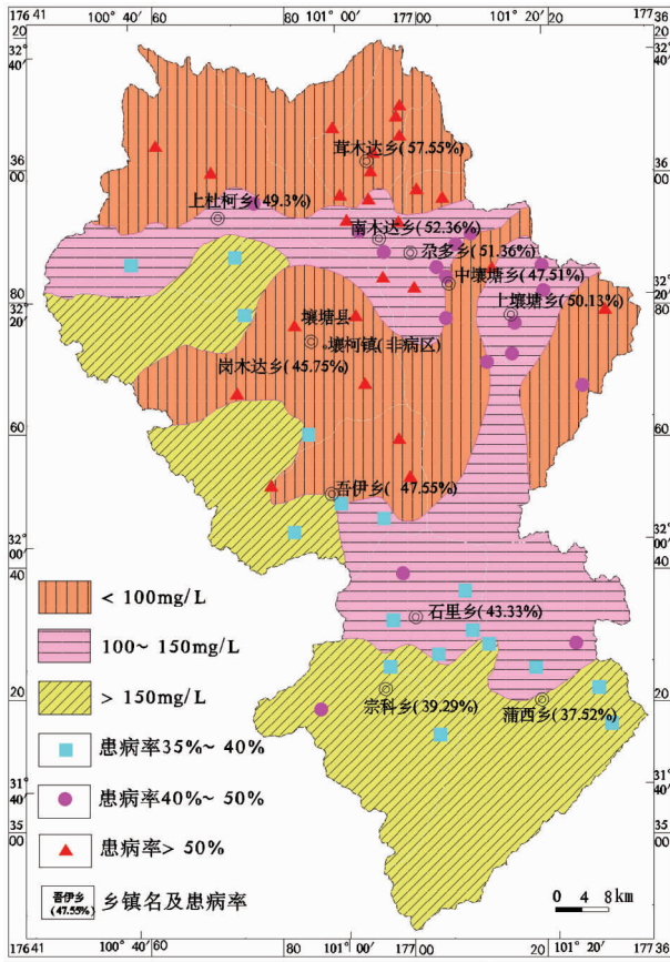
图 1 大骨节病病情与矿化度关系略图
