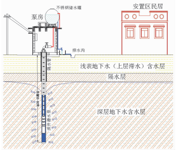
图 2 探采结合示范井开采模式图
