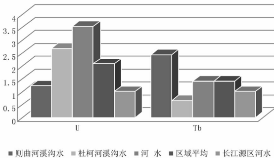
图8 放射性元素不同流域比较
