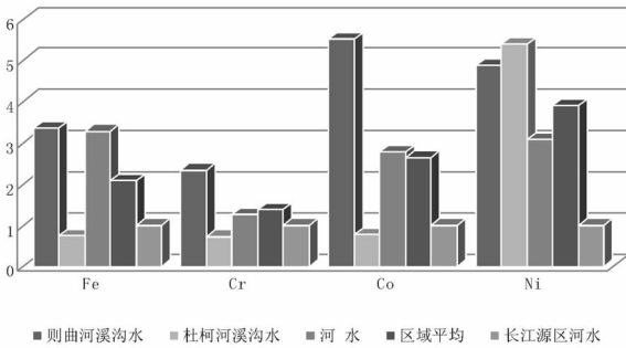
图 2 铁族元素以及亲铜元素流域比较
