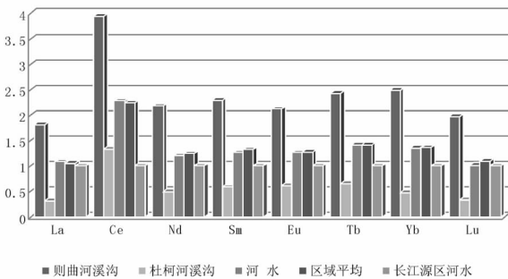
图 4 稀土元素不同流域比较
