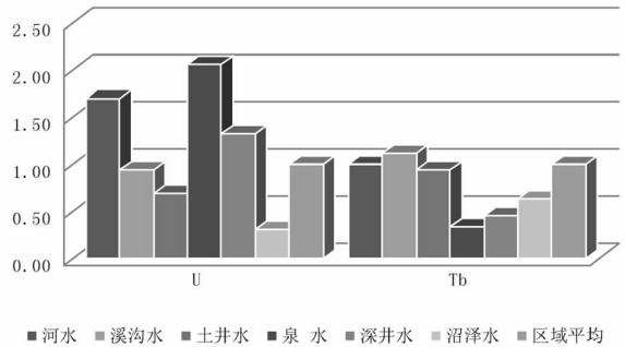
图9 放射性元素不同水源类型比较
