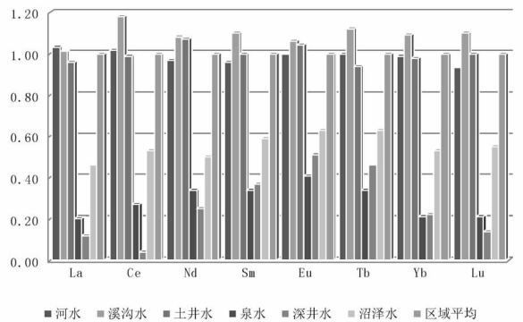
图 5 稀土元素不同类型水源比较
