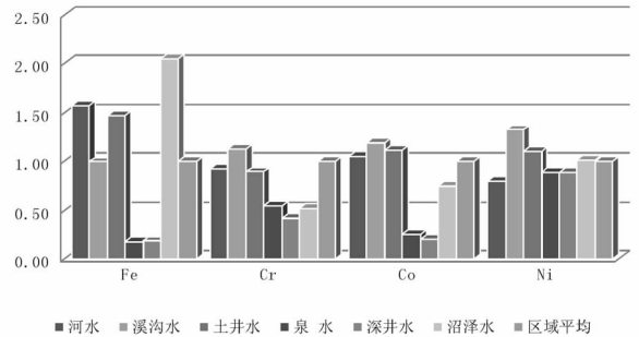
图 3 铁族元素以及亲铜元素不同类型水源比较
