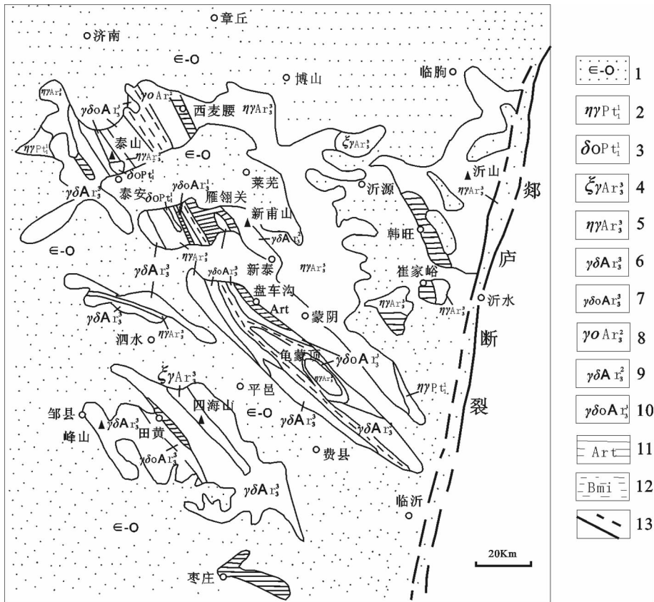
图1 鲁西地区简化地质图(据王世进,1990 [5] ,修改补充)
