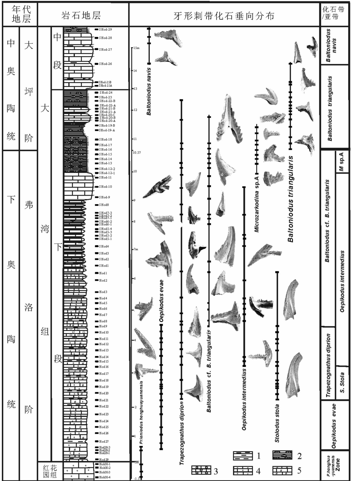
图 2 湖北宜昌黄花场剖面红花园组顶部—大湾组下段牙形石分带和属种分布
