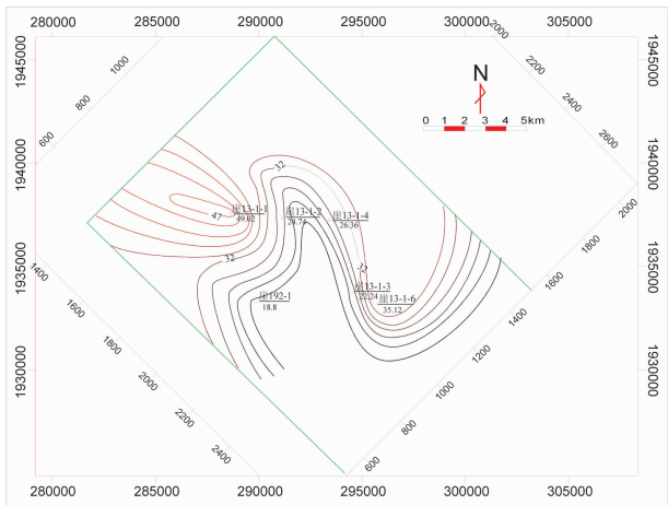
图7 陵三段不稳定重矿物含量等值线图
