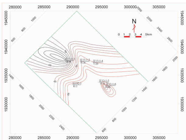
图5 陵三段稳定重矿物含量等值线图
