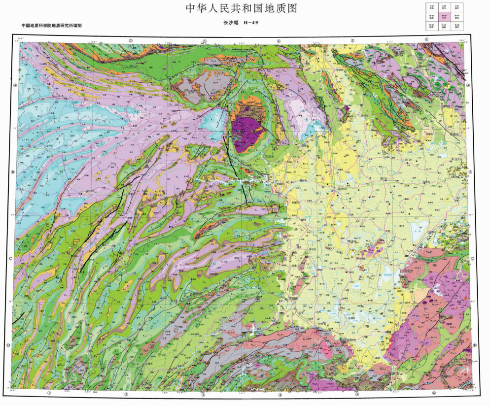
图 4 1:100 万长沙幅(H-49)地质图
