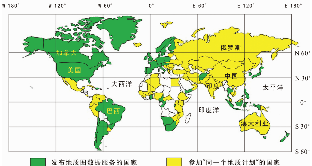
图 1 “OneGeology 计划”参与国家(底图据 www.onegeology.org )
