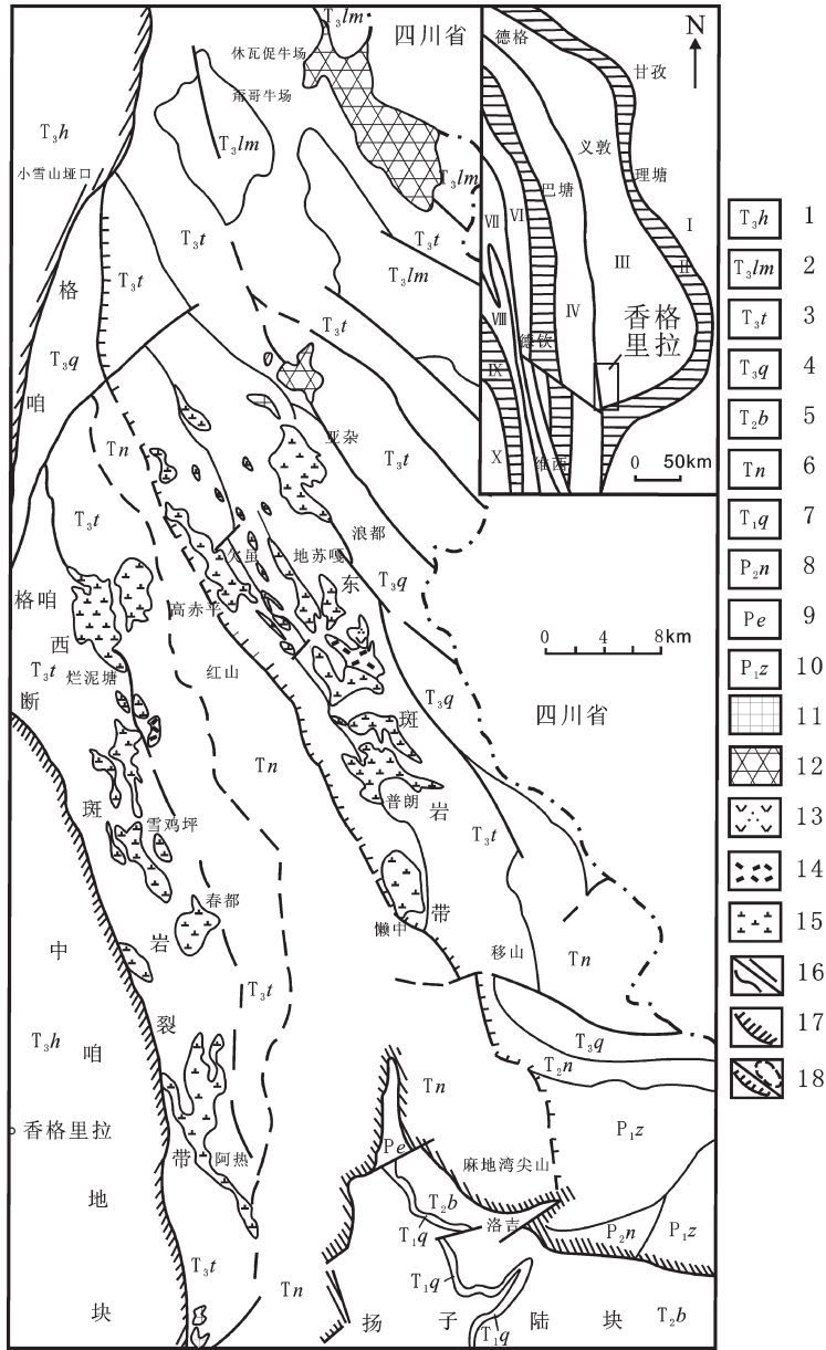
图1 香格里拉地区侵入岩分布略图(底图据文献[5],有修改)
