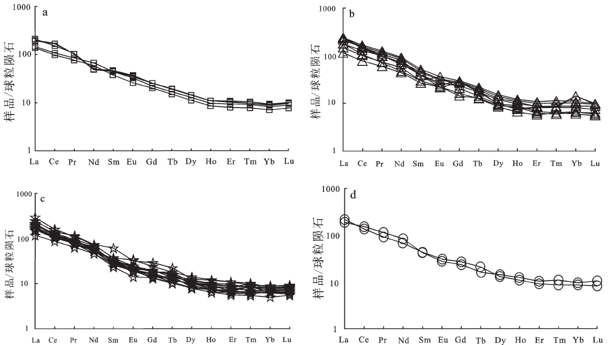
图 3 稀土配分曲线
