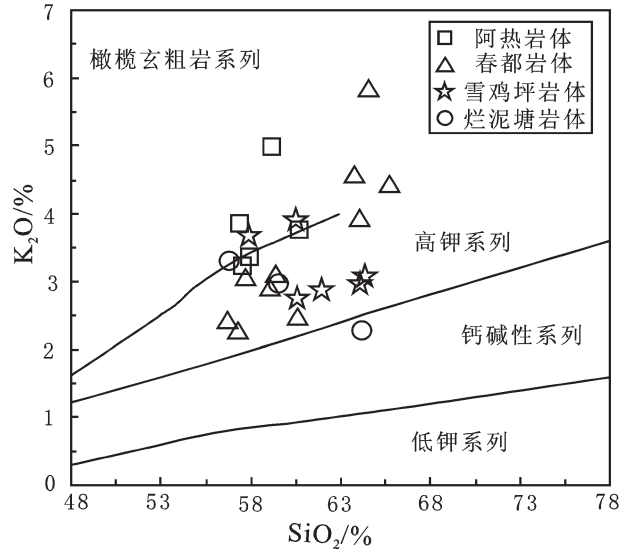
图 2 SiO 2 -K 2 O 图解(底图据 [23] ) Fig.2 Diagram of K 2 O versus SiO 2 (after [23] )
