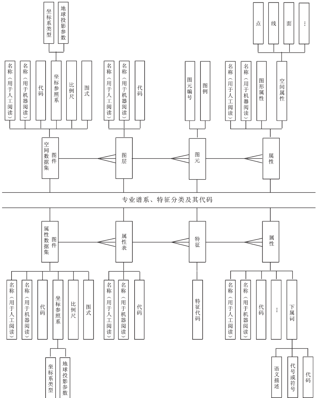
图4 图件数据模型的概念框架
