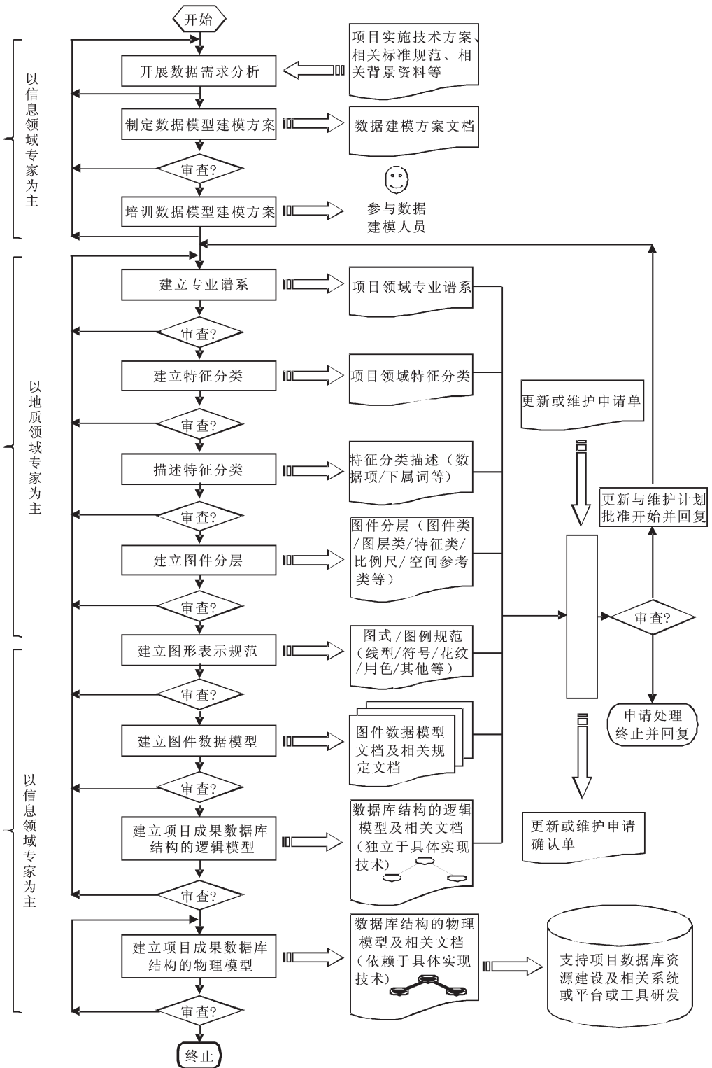
图 1 数据模型研制流程
