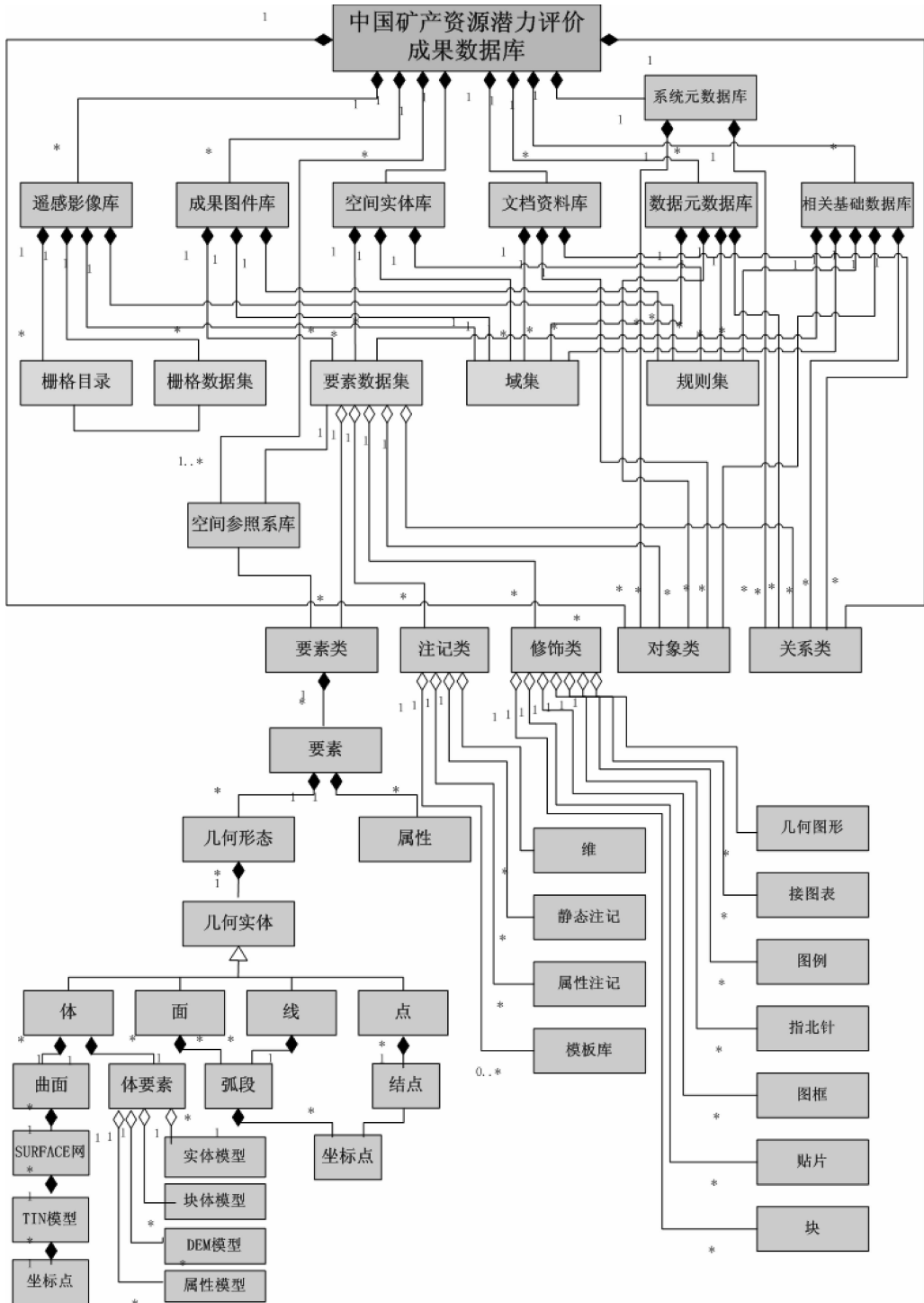
图 8 中国矿产资源潜力评价数据库内容基本结构模型
