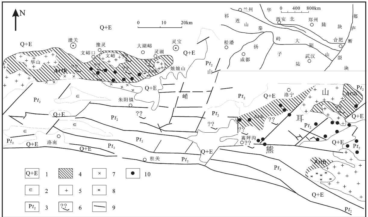
图 3 小秦岭地区地质简图(据文献[30]修改)
