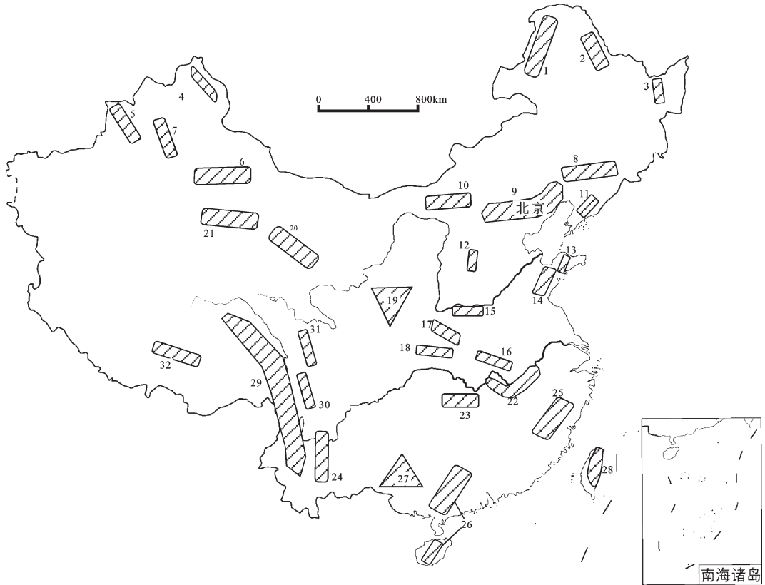
图 1 中国金矿矿集区分布图(编号见表 2)
