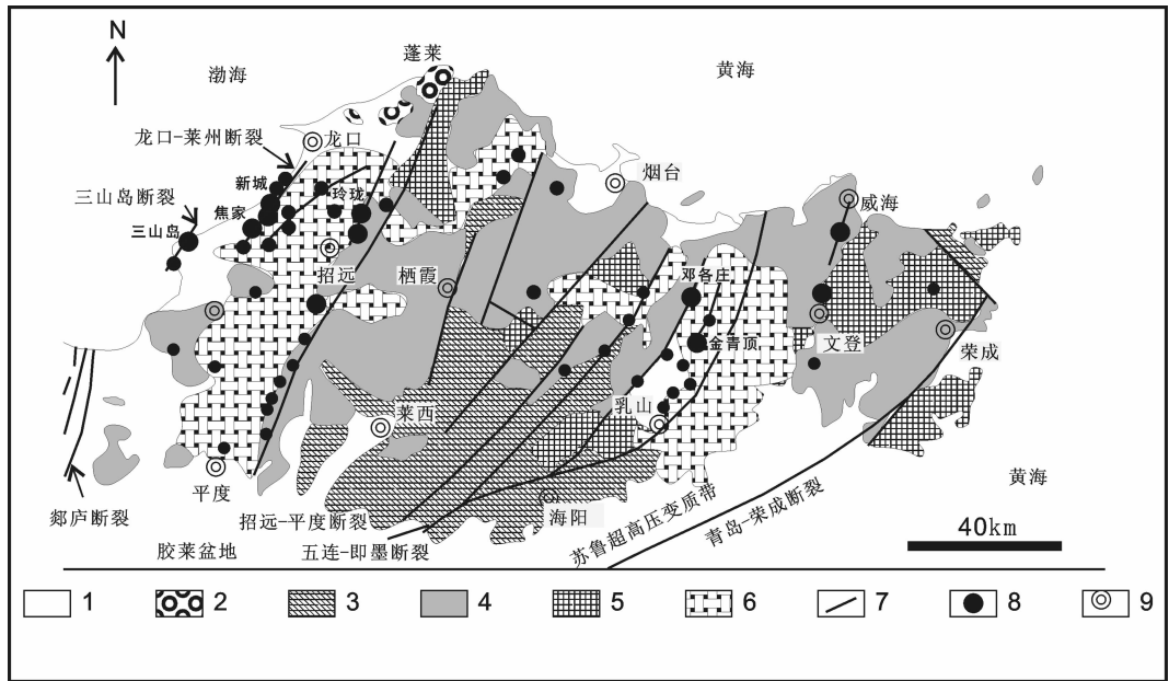
图2 胶东矿集区金矿地质简图(据文献[26])
