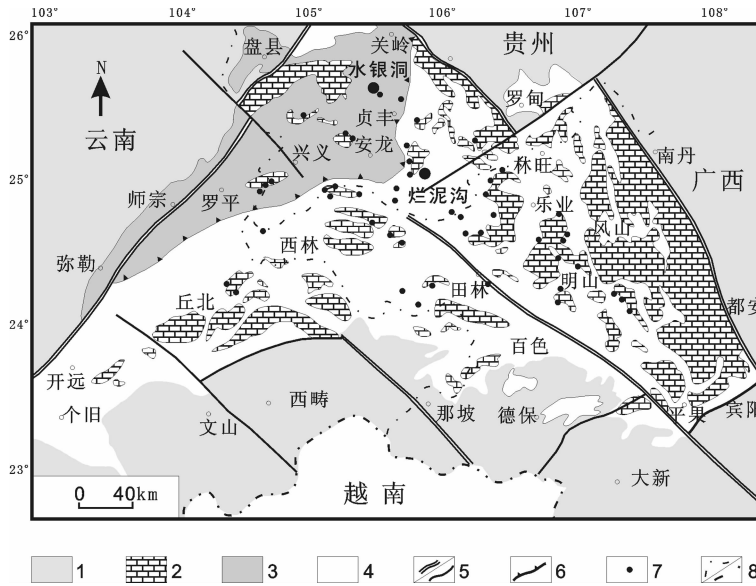
图 4 滇黔桂金矿集区地质略图
