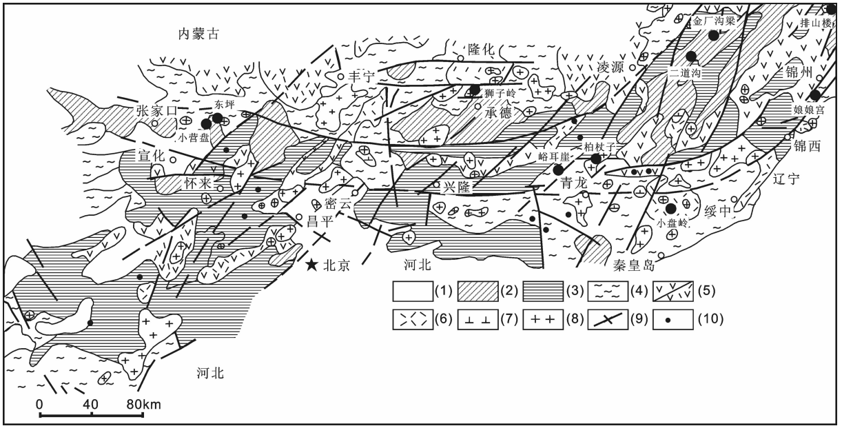
图5 燕辽地区金矿集区地质简图(据文献[49]修改)
