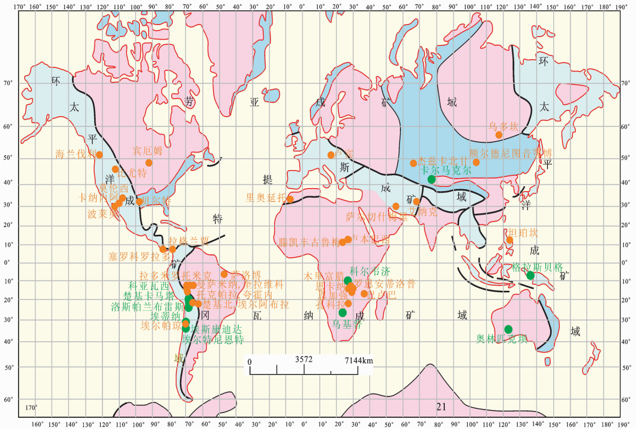
图1 超大型-特大型铜矿床分布略图
