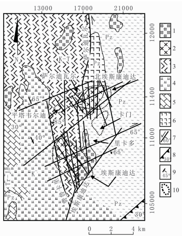
图 3 埃斯康迪达铜矿床区域地质略图 [53]
