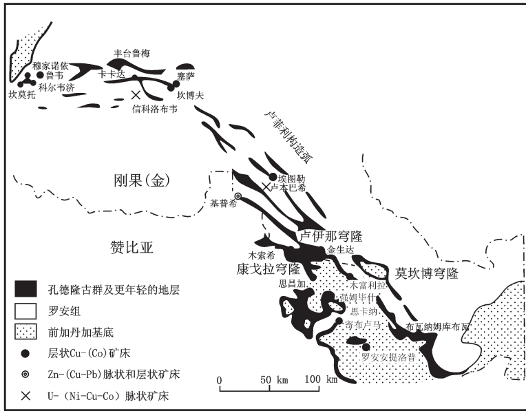
图5 中非铜矿带区域地质略图 [38]
