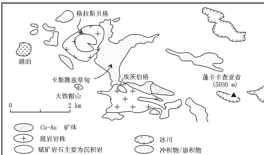
图 4 印度尼西亚格拉斯贝格地区铜金矿床分布略图 [54]
