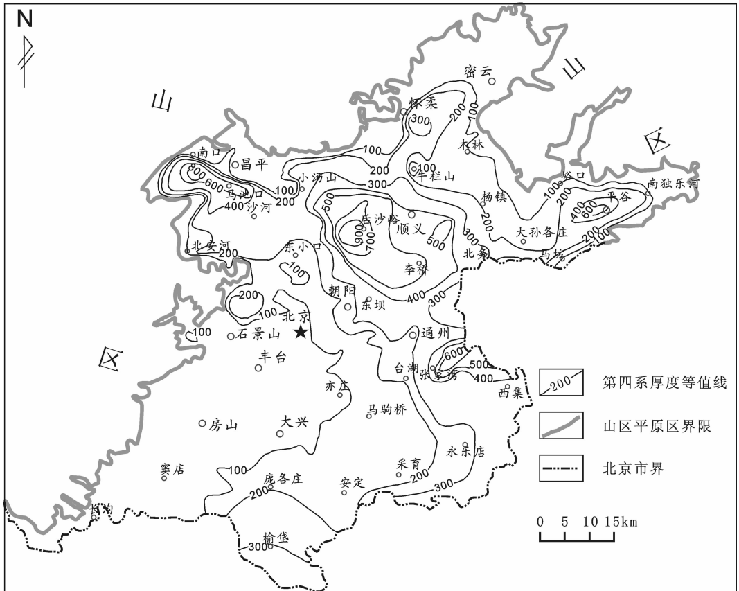
图 2 北京平原第四系等厚度图
