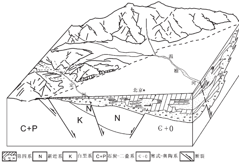
图 1 北京平原地质构造与地貌示意图
