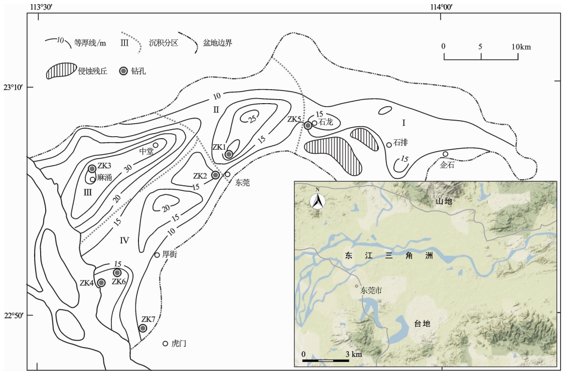
图 1 东江三角洲地貌(底图据 Google 地图)、第四系等厚线 [15] 及钻孔位置
