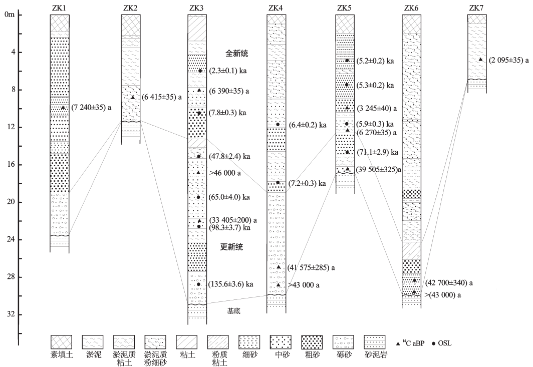
图 2 东江三角洲第四系钻孔剖面年代对比
