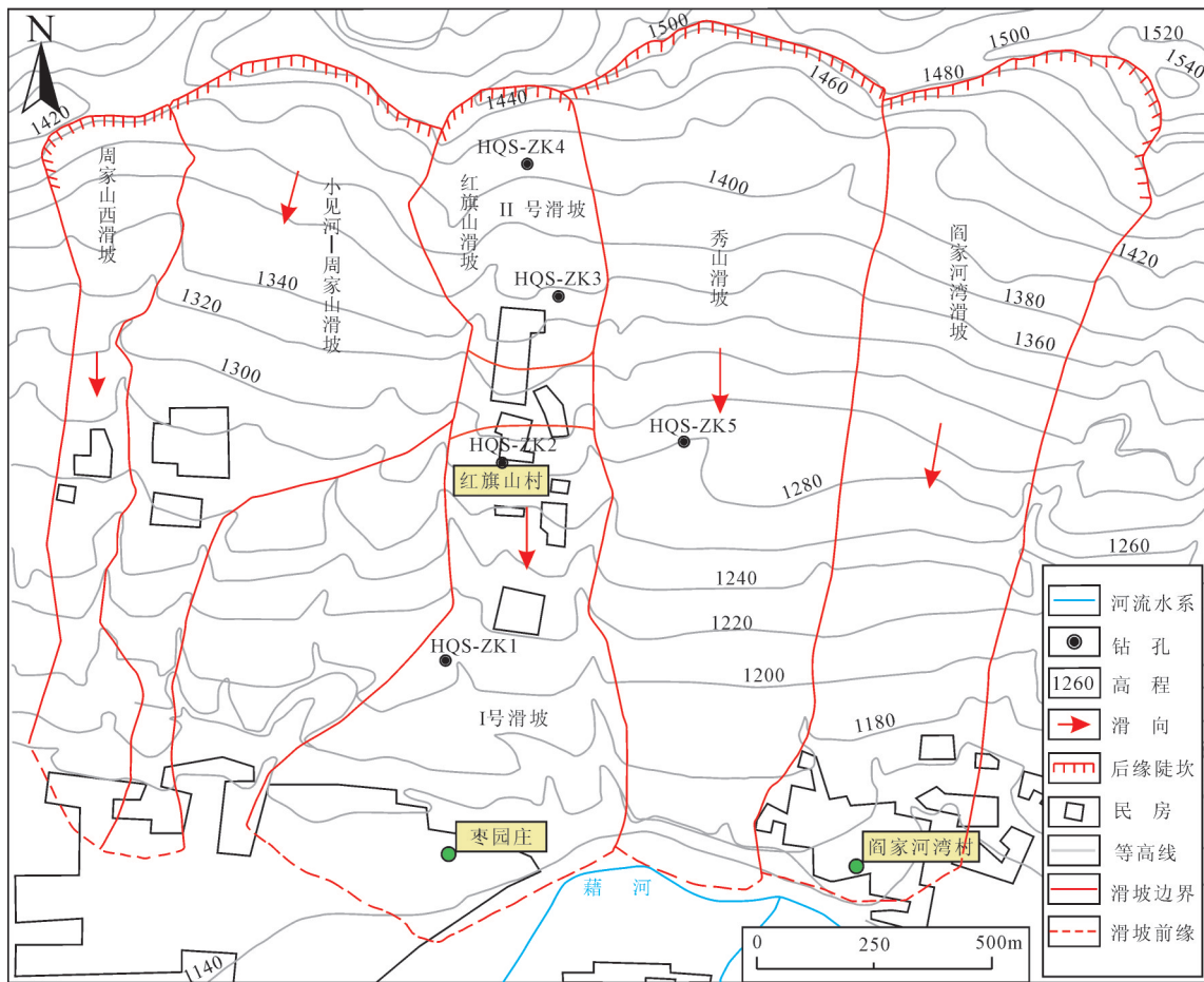
图2 天水市秦州区北山红旗山地震滑坡群平面图
