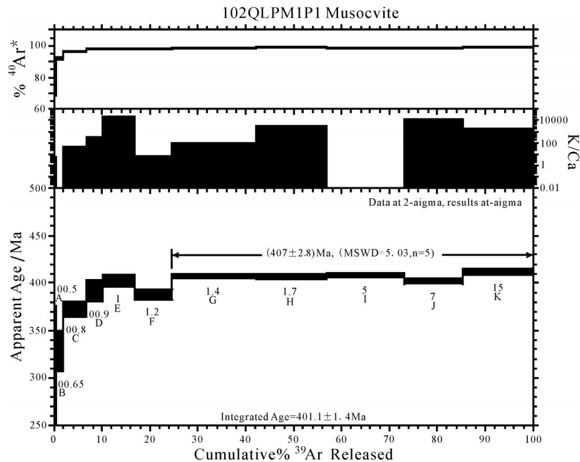
图1 群力铁多金属矿床砂卡岩矿石中白云母的 40 Ar/ 39 Ar阶段升温年龄谱图
