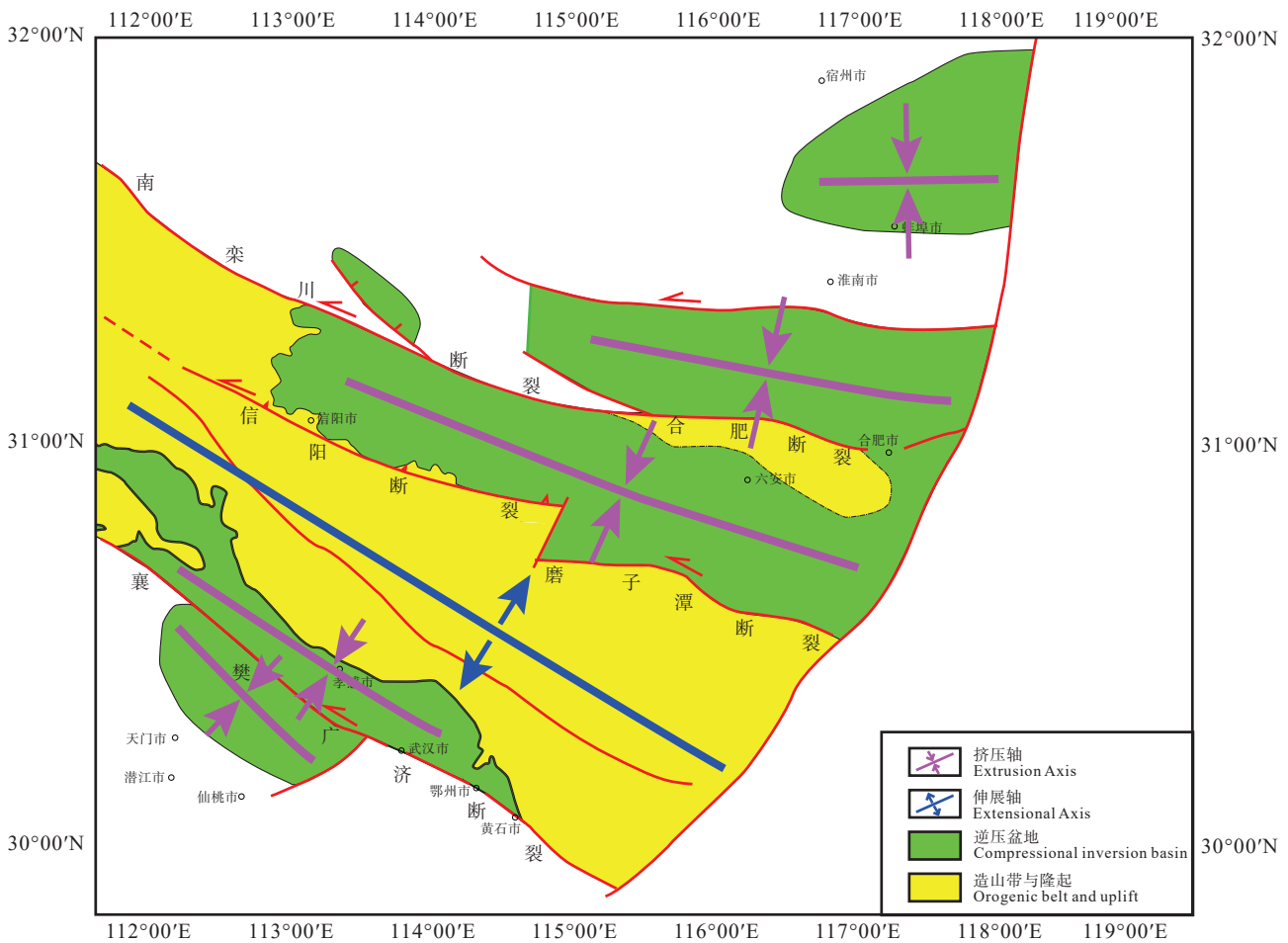
图 10 中国秦岭大别造山带与南华北盆地中、新生代盆山正、负构造反转体系图
