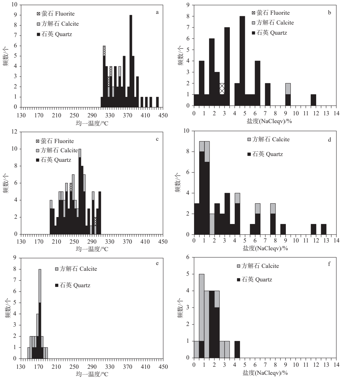
图 6 二道河铅锌银矿流体包裹体均一温度与盐度分布直方图
