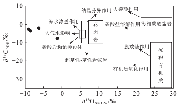
图7 二道河铅锌银多金属矿床方解石的C、O同位素值分布(改自刘家军等, 2004)
