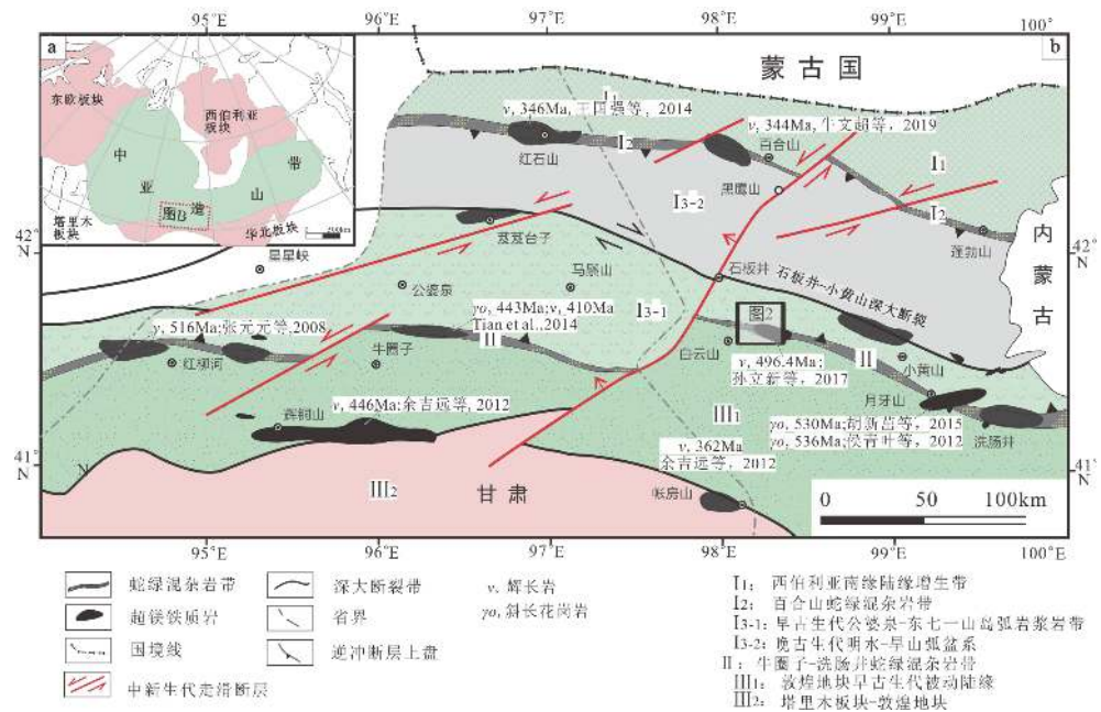
图 1 内蒙古北山造山带大地构造位置图 (a) 及北山地区蛇绿构造混杂岩带时空分布略图 (b) (据杨合群等, 2010; Xiao WJ et al., 2010; 牛文超等, 2019 改编)
