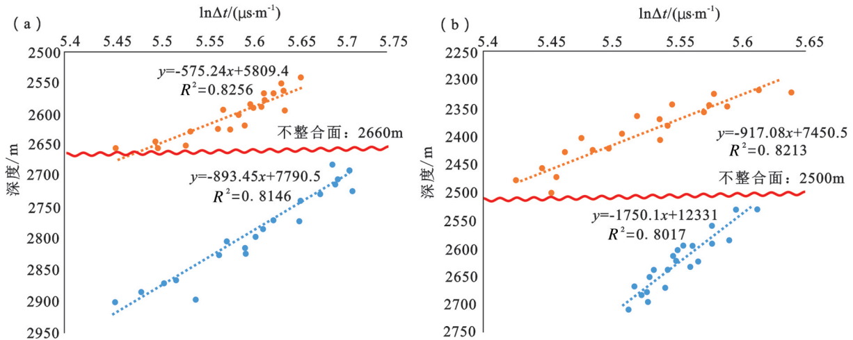
图4 临河拗陷声波时差法确定不整合面 a—吉参1井; b—松探1井
