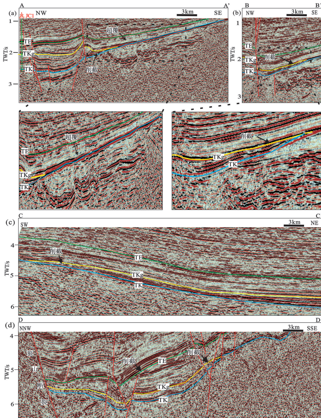
图5 吉参1井过井地震标定及临河拗陷典型地震剖面(位置见图6,说明见正文)
