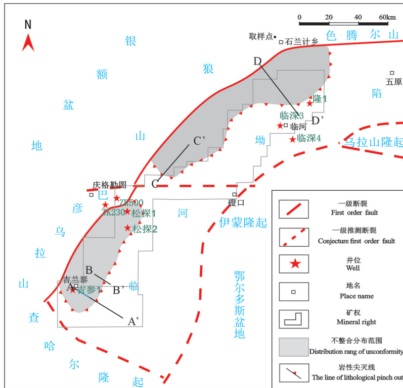
图6 临河拗陷下白垩统内部不整合平面分布图
