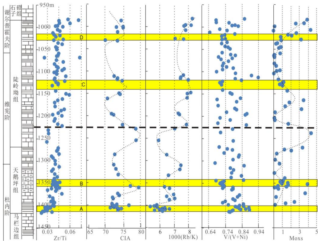
图 5 湘中下石炭统物源、盐度, 气候和生产力指标变化曲线(图例同图 3)
