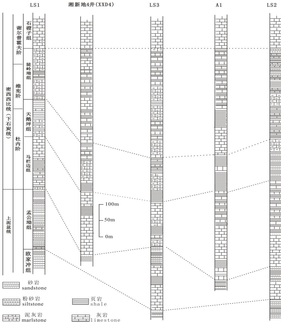
图 3 湘中涟源凹陷上泥盆统一下石炭统划分对比图(钻井位置见图 1)
