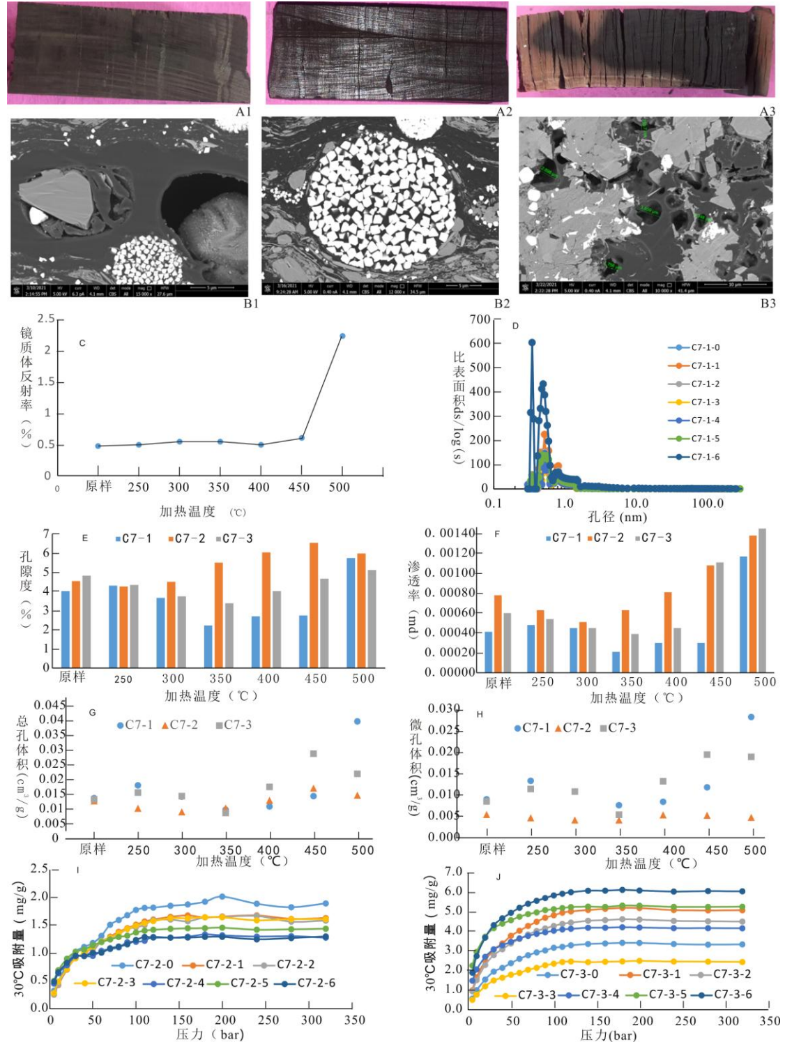
图6 不同模拟温度下页岩储层的物性和含气性特点
