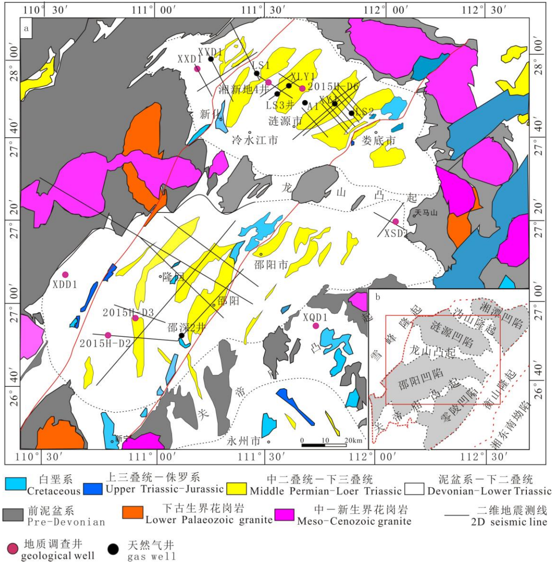
图 1 湘中坳陷地质简图和页岩气勘探程度图
