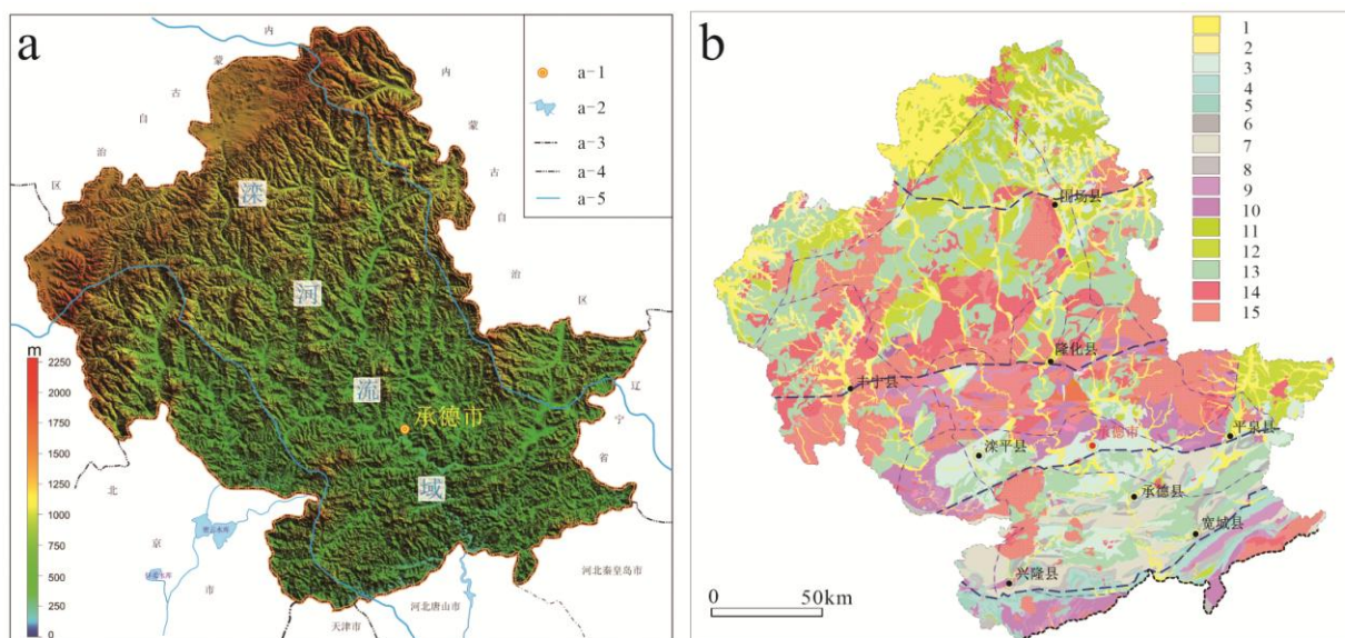
图1 承德市地形地貌图 (a) 及承德市地质建造图 (b) (引自卫晓锋等, 2020)
