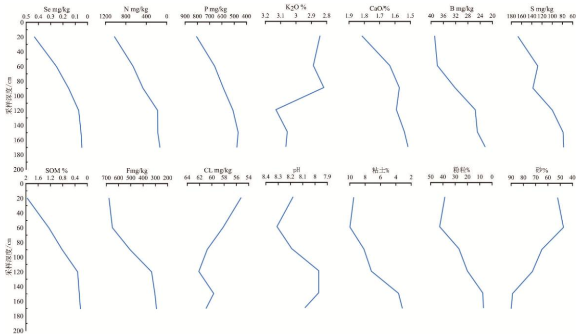
图 5 承德市南部 (B 区) 河道沉积型土壤不同元素的垂向剖面测量值
