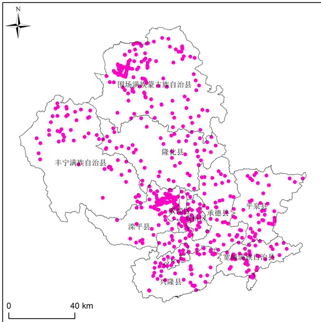
图 2 承德市表层土壤采样点分布图
