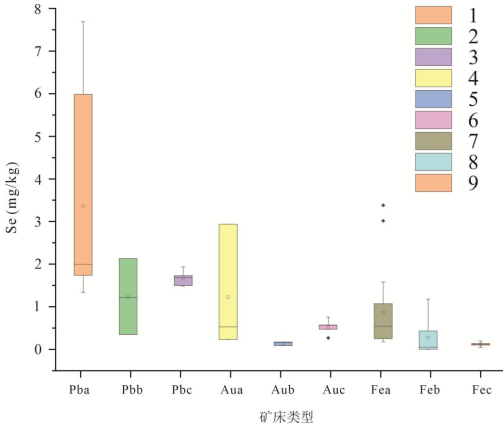
图 4 承德市主要矿床类型的硒含量等级图
