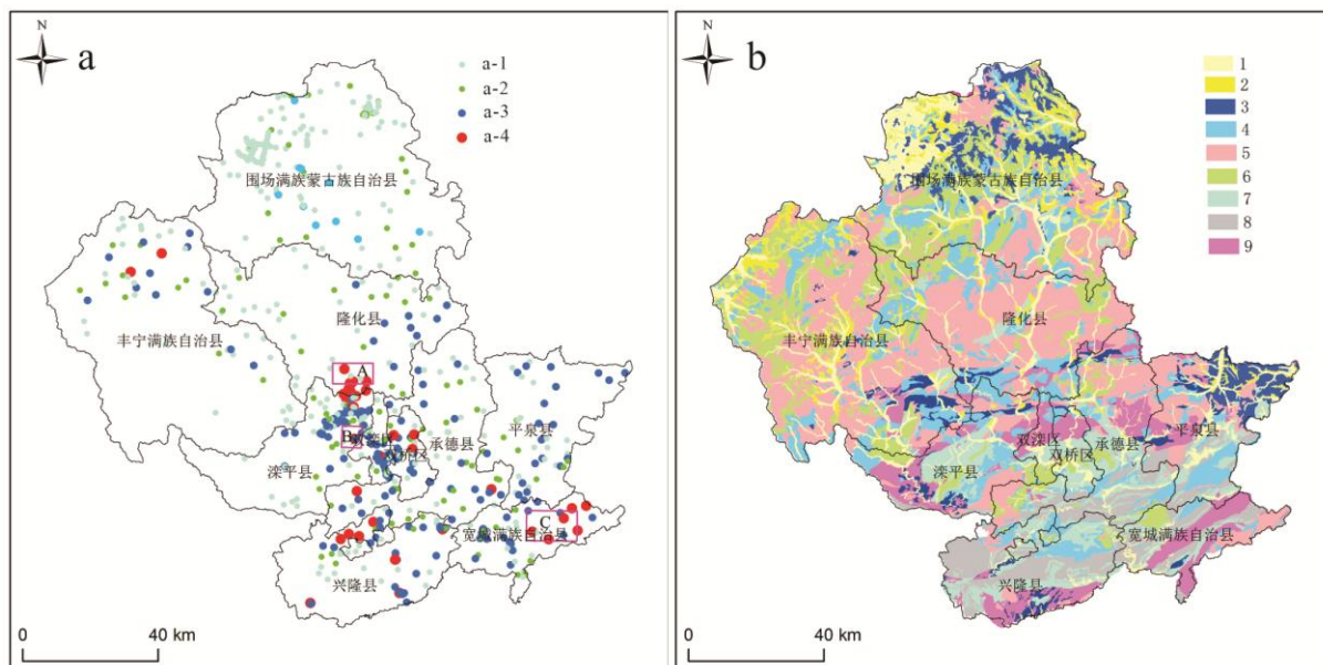
图3 承德市表层土壤富硒等级图 (a) 和成土母质分布图 (b)
