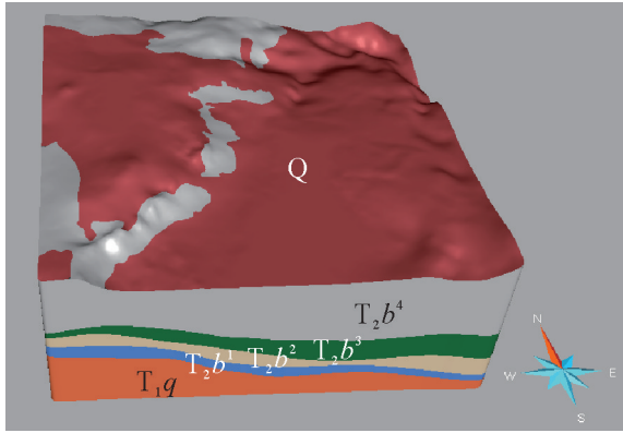
图3 万铜山矿区地层界面模型
