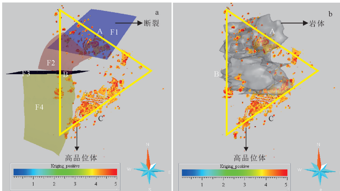
图10 断裂(a)、岩体(b)(70%透明度)与金高品位体(品位>4 g/t)的关系
