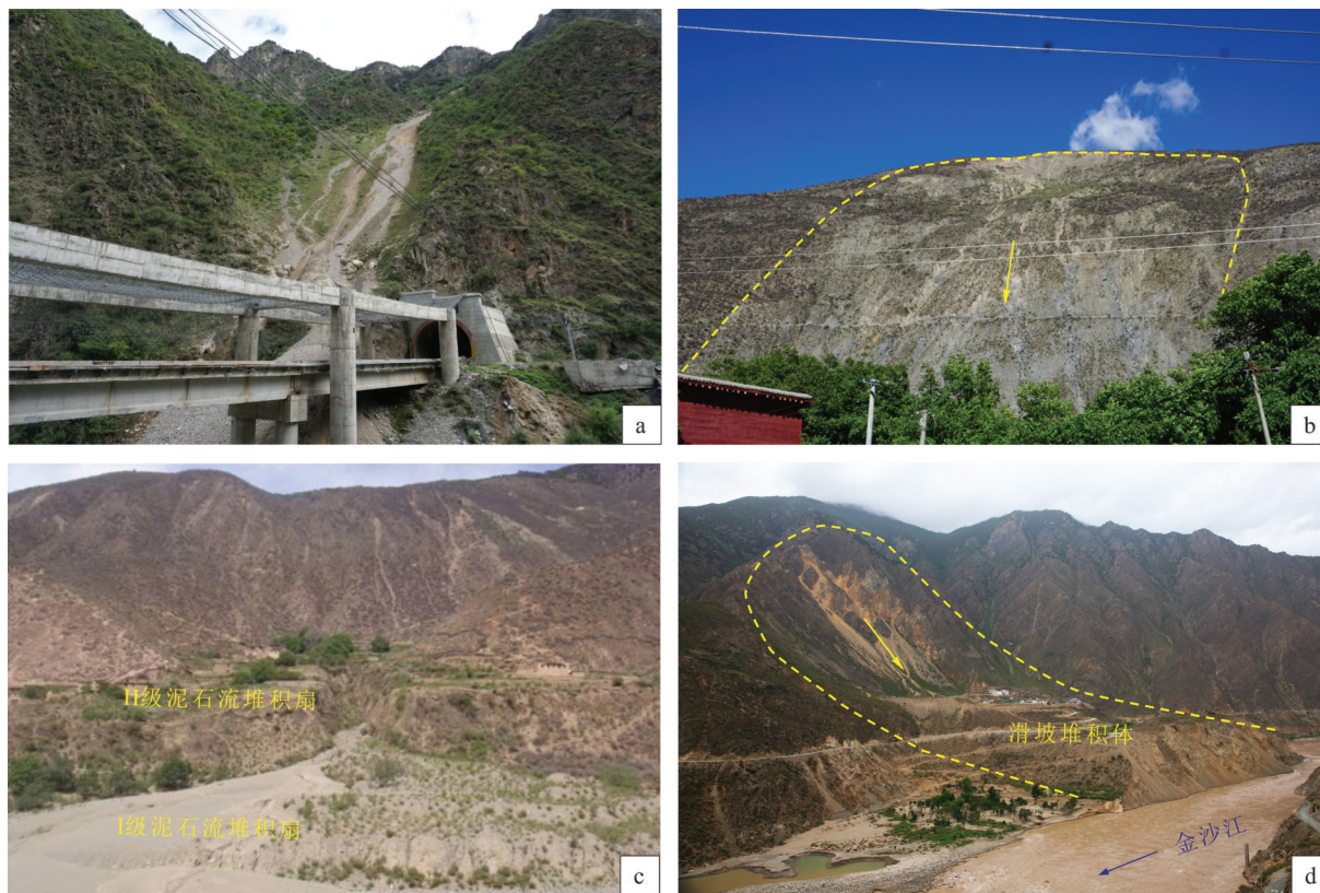
图5 巴塘断裂带典型地质灾害实例
