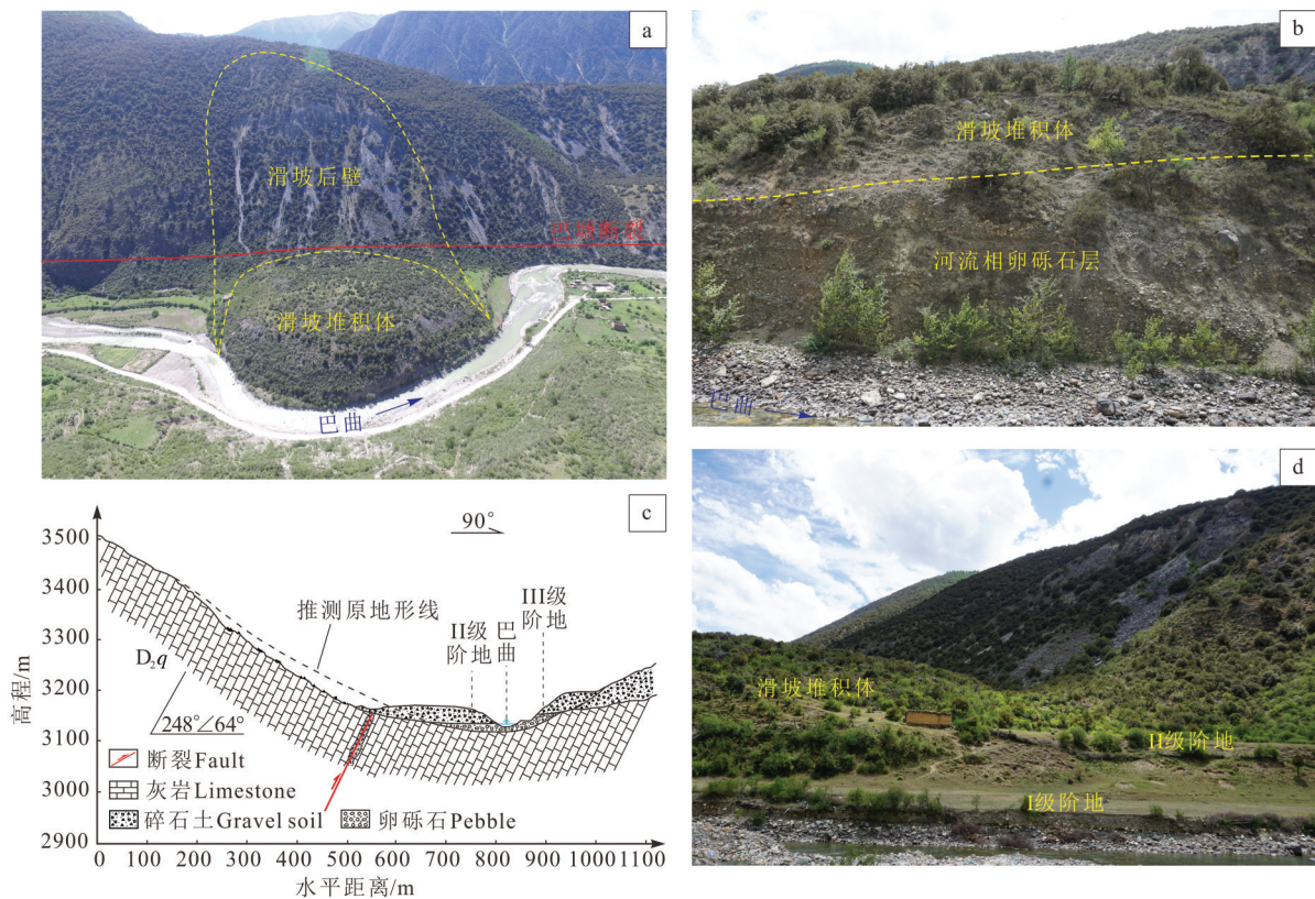
图9 巴塘郎多二村滑坡发育特征
