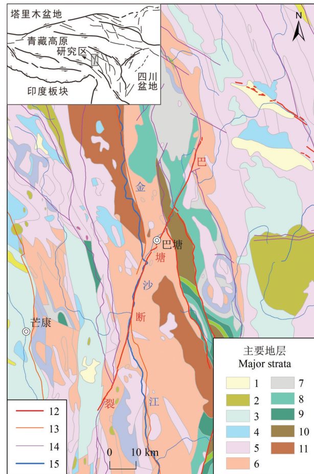
图 1 巴塘断裂带地质背景图
