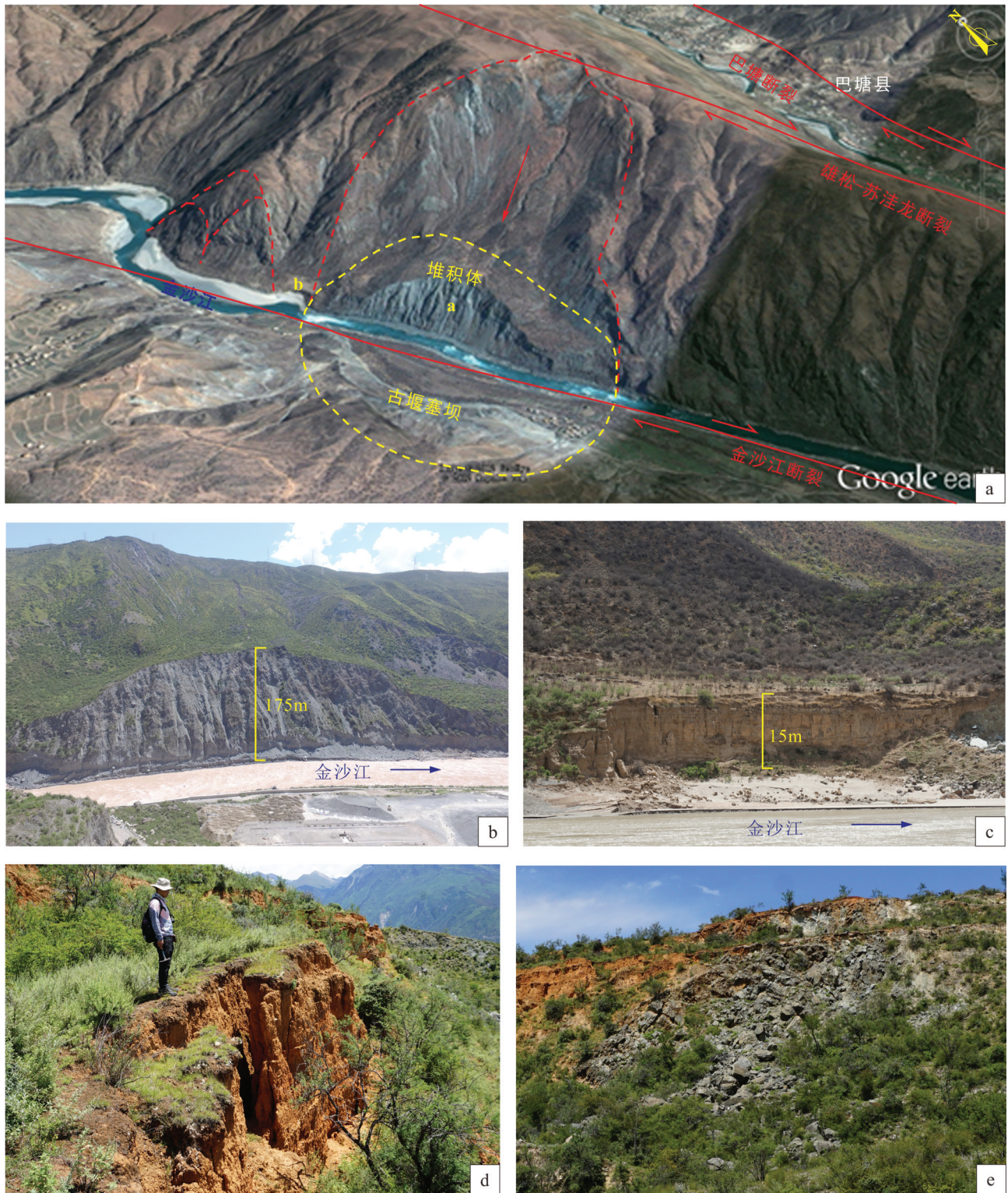
图8 巴塘特米滑坡发育特征
