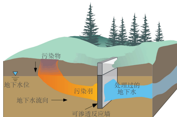
图6 地下水污染可渗透性反应墙技术示意图(USEPA, 1998)
