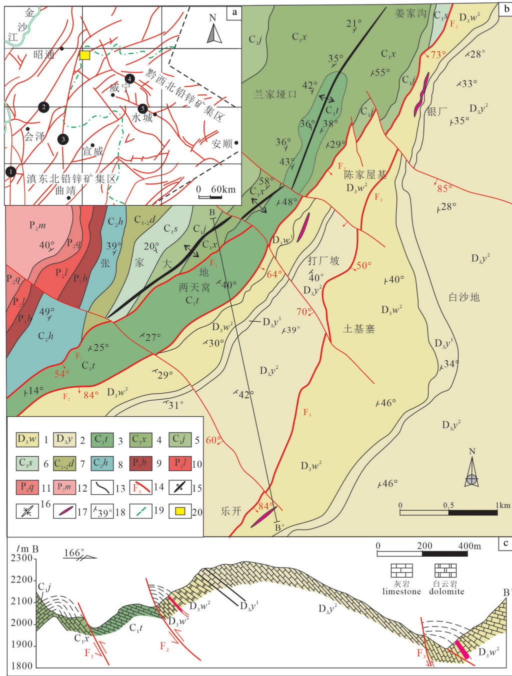
图1 a—乐开铅锌矿床地质简图;b—川滇黔区域地质图(据柳贺昌, 1995修改);c—矿区BB'实测地质剖面图 1—泥盆系望城坡组; 2—泥盆系尧梭组; 3—石炭系汤耙沟组; 4—石炭系祥摆组; 5—石炭系旧司组; 6—石炭系上司组; 7—石炭系大浦组; 8—石炭系黄龙组; 9—二叠系包磨山组; 10—二叠系梁山组; 11—二叠系栖霞组; 12—二叠系茅口组; 13—地层界线; 14—断裂及编号; 15—背斜; 16—向斜; 17—矿体; 18—产状; 19—省界; 20—研究区; ①—小江断裂带; ②—会泽—牛街断裂带; ③—昭通—曲靖隐伏断裂带; ④—垭都—蟒洞断裂带; ⑤—威宁—水城断裂带
