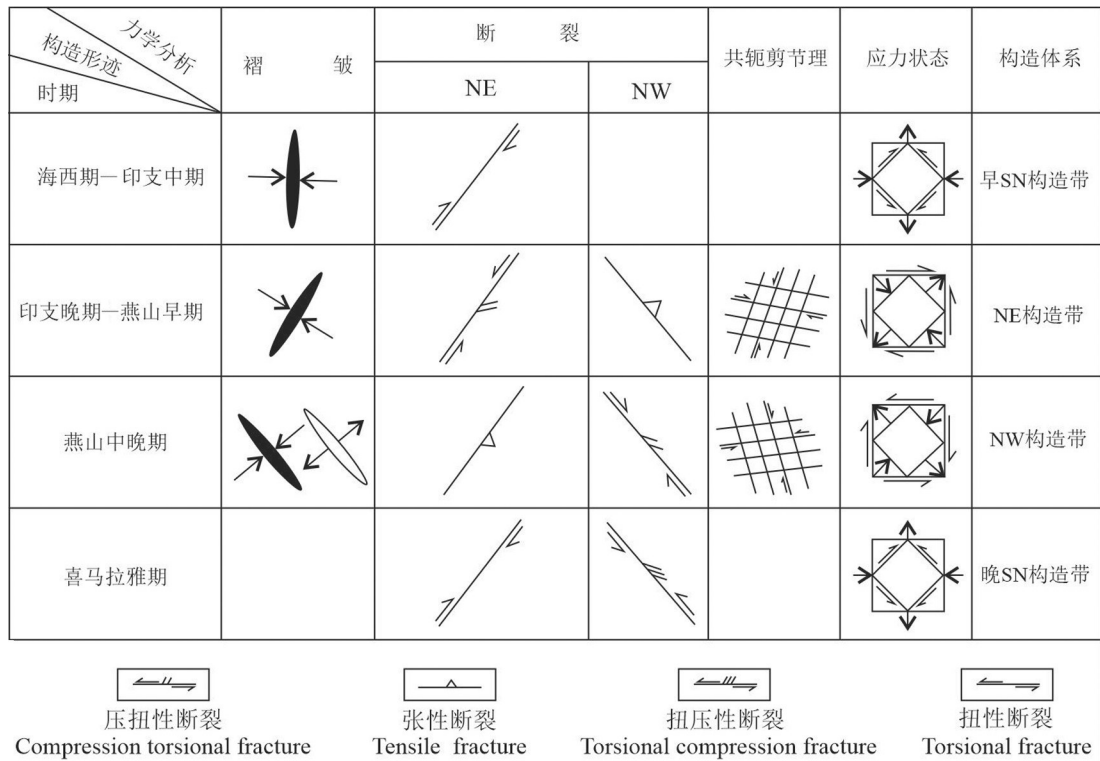
图10 乐开铅锌矿区构造体系成生发展及其演化图解
