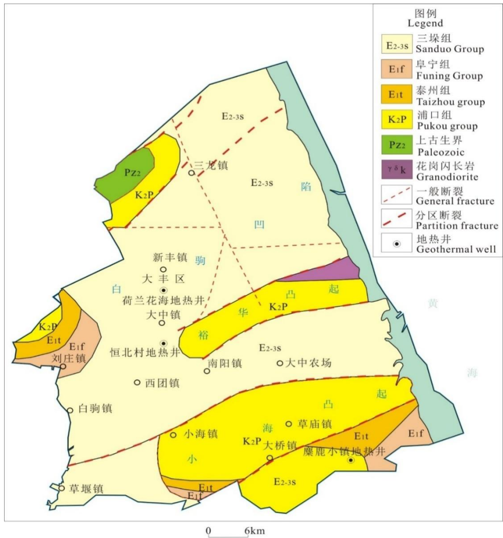
图2 大丰区地质构造图 Fig.2 Geological structure map of Dafeng District
