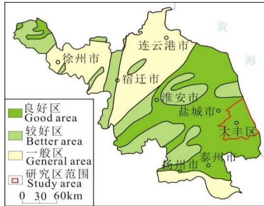
图 1 大丰区区域地热地质条件分区图
