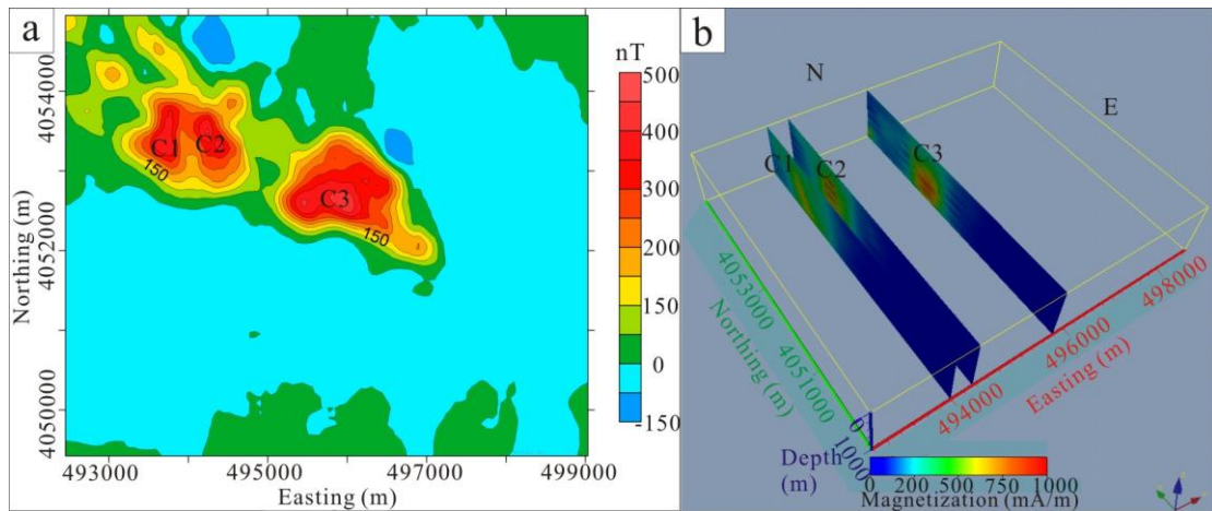
图 11 开木棋岩体地面磁测数据化极图 (a) 和三维磁化率反演图 (b) . C1、C2 和 C3 为磁异常编号。
