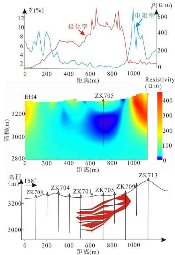
图 12 夏日哈木 7 号线激电中梯和高频大地电磁测深异常图(宋梦馨, 2015)
