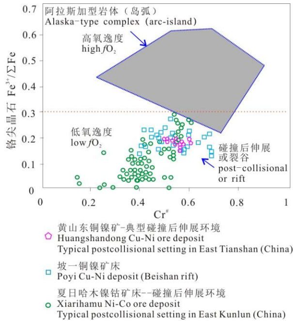
图4 夏日哈木岩体氧逸度与岛弧阿拉斯加型岩体氧逸度的对比(Liu et al., 2018) 阿拉斯加范围和夏日哈木超大型 Ni-Co 矿床铬尖晶石来源于(Liu et al., 2018), 黄山东 Cu-Ni 矿床铬尖晶石据(傅飘儿, 2012), 坡一 Cu-Ni 矿床铬尖晶石据(吴建亮等, 2018)
