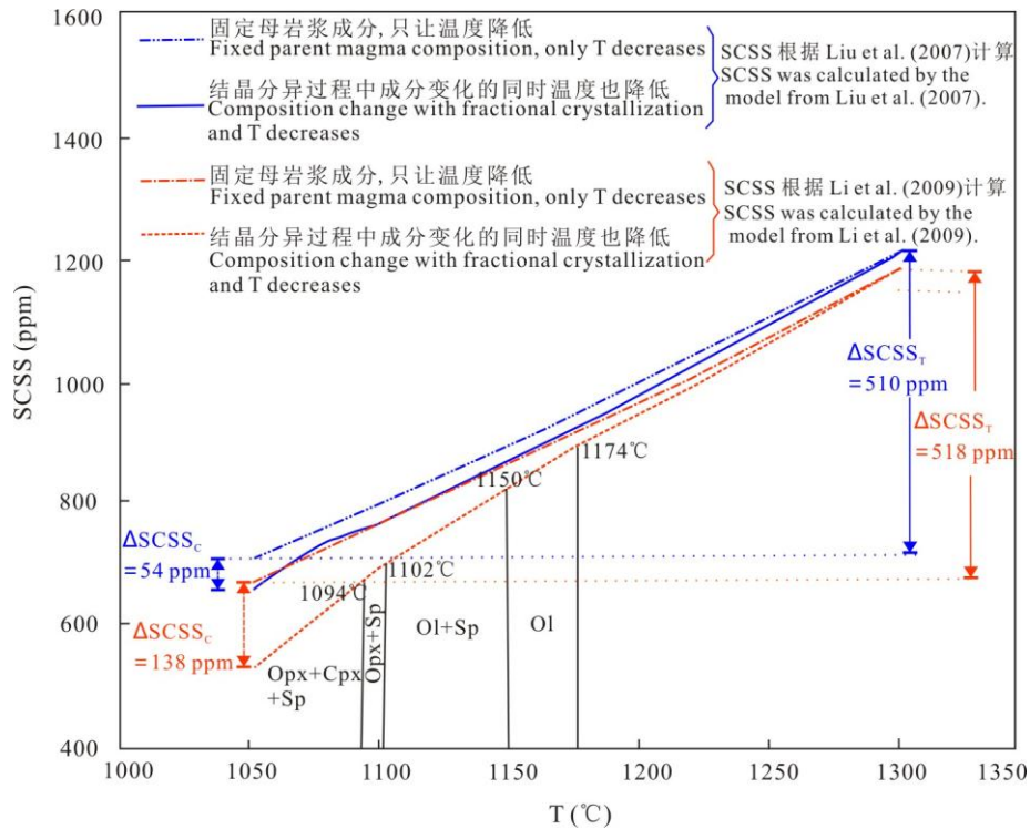
图 5 结晶过程中 SCSS 变化情况的定量模拟(Liu et al., 2018)
