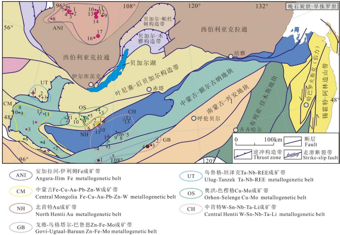
图9 区域晚石炭世-早侏罗世主要成矿带 (成矿带划分据表1中参考文献)
