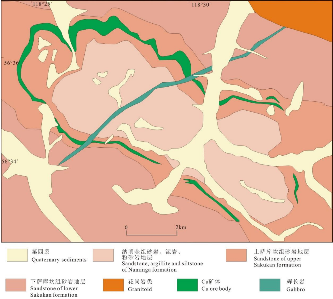
图 4 乌多坎铜矿床地质图 (据 Gongalsky and Krivolutskaya, 2019)
