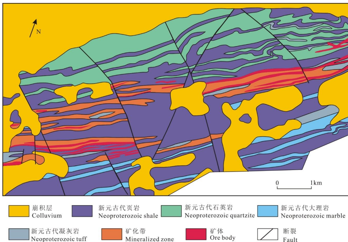
图 5 霍洛德宁铅锌矿床地质简图 (据 Добровольская and Ерёмин, 2010)
