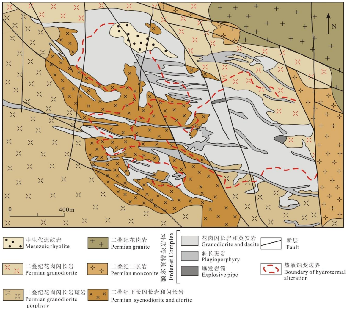
图 10 额尔登特铜钼矿床地质简图 (据 Sotnikov et al., 2005)
