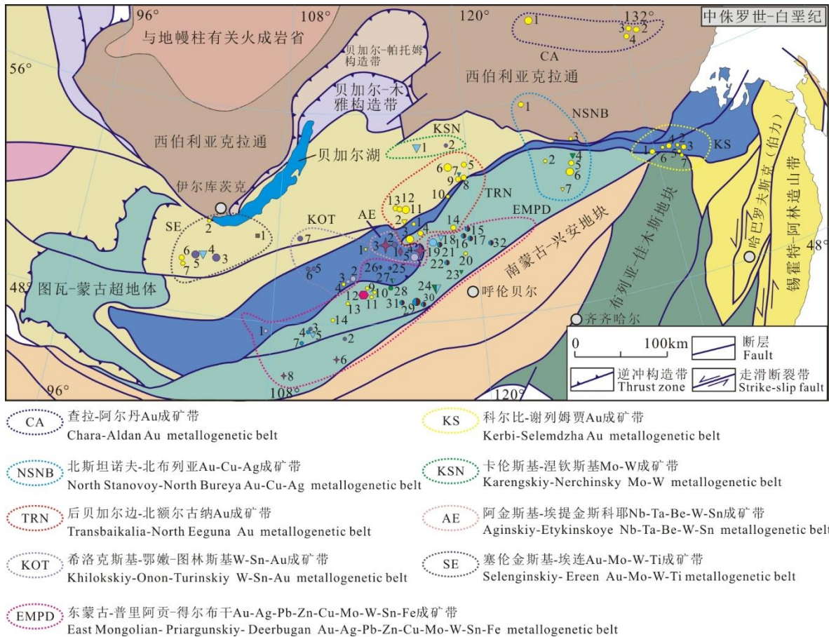
图 11 区域中侏罗世-白垩纪主要成矿带（成矿带划分据表 1 中参考文献）
