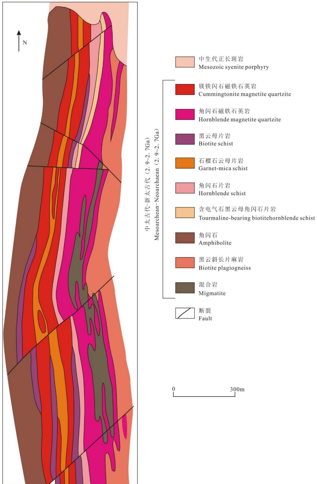
图 2 塔林纳赫铁矿床地质简图 (据 Petrov et al., 2017)
