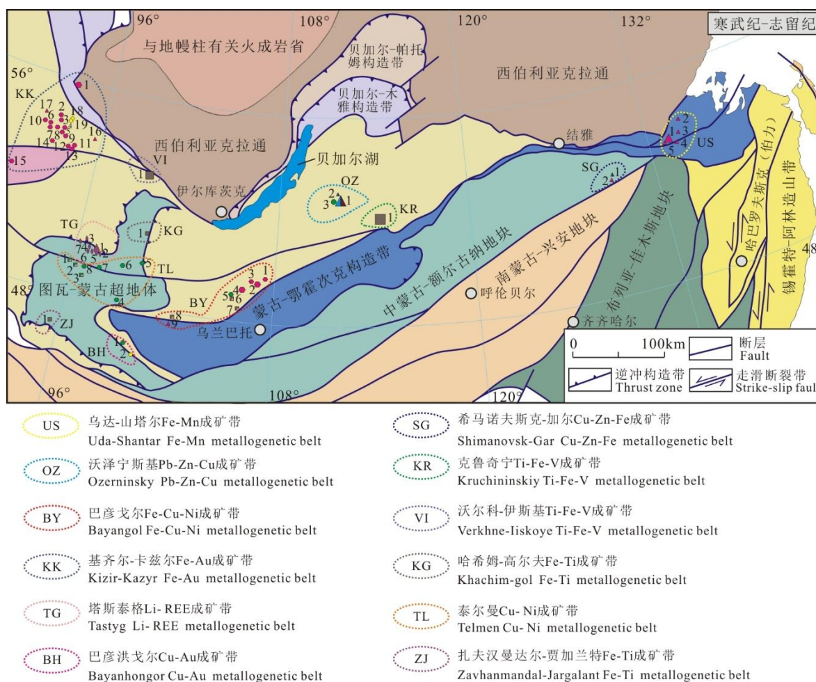
图 6 区域寒武纪-志留纪主要成矿带（成矿带划分据表 1 中参考文献）
