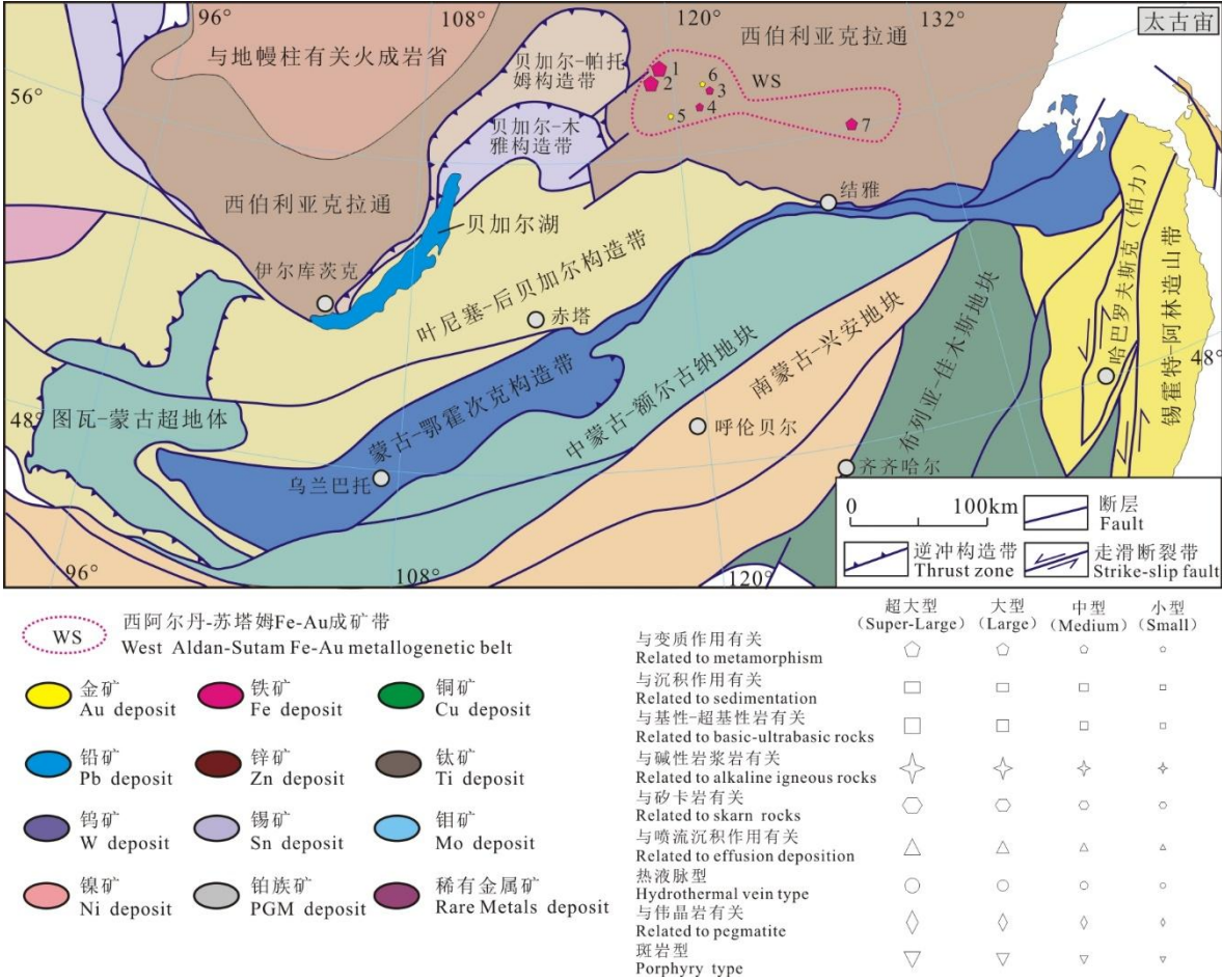
图 1 区域大地构造划分和太古宙主要成矿带 (据 Parfenov et al., 2001; Badarch et al., 2002; Nokleberg, 2010;成矿带划分据表 1 中参考文献)
