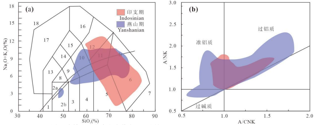
图 3 南岭成矿带中段岩浆岩 TAS 图解 (a) 和 A/NK—A/CNK 图解 (b)
