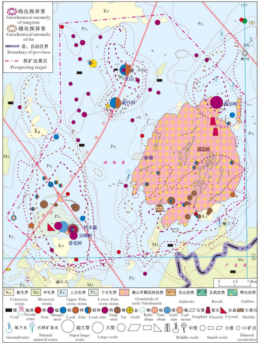
图 8 南岭中段骑田岭钨锡钼铋铅锌铜金稀土萤石找矿远景区矿产地质简图
