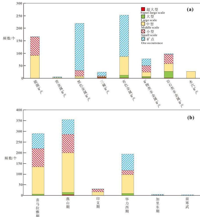
图 6 南岭成矿带中段不同矿种 (a) 和不同世代 (b) 矿产规模柱状图
