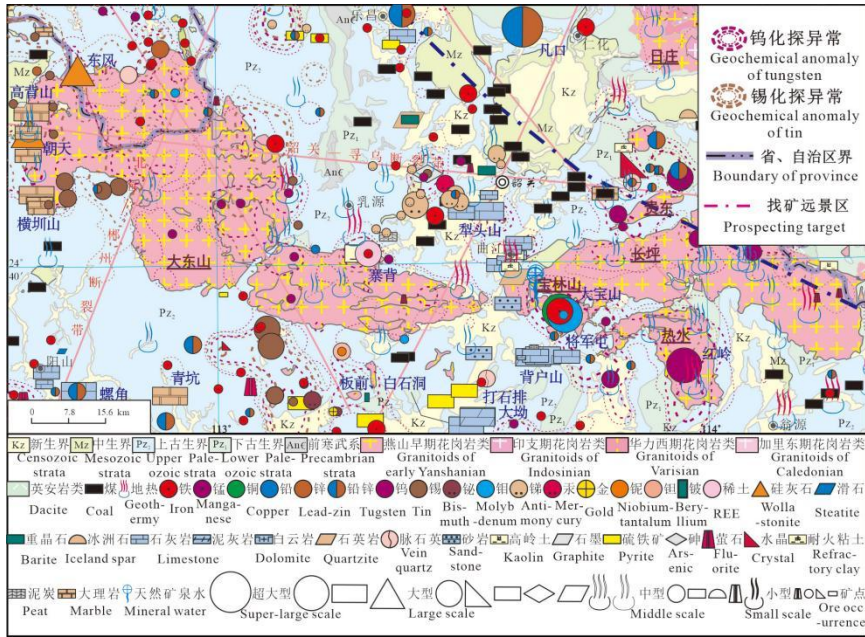
图9 南岭中段乐昌—韶关—翁源钨锡铜铅锌铀稀土找矿远景区矿产地质简图
