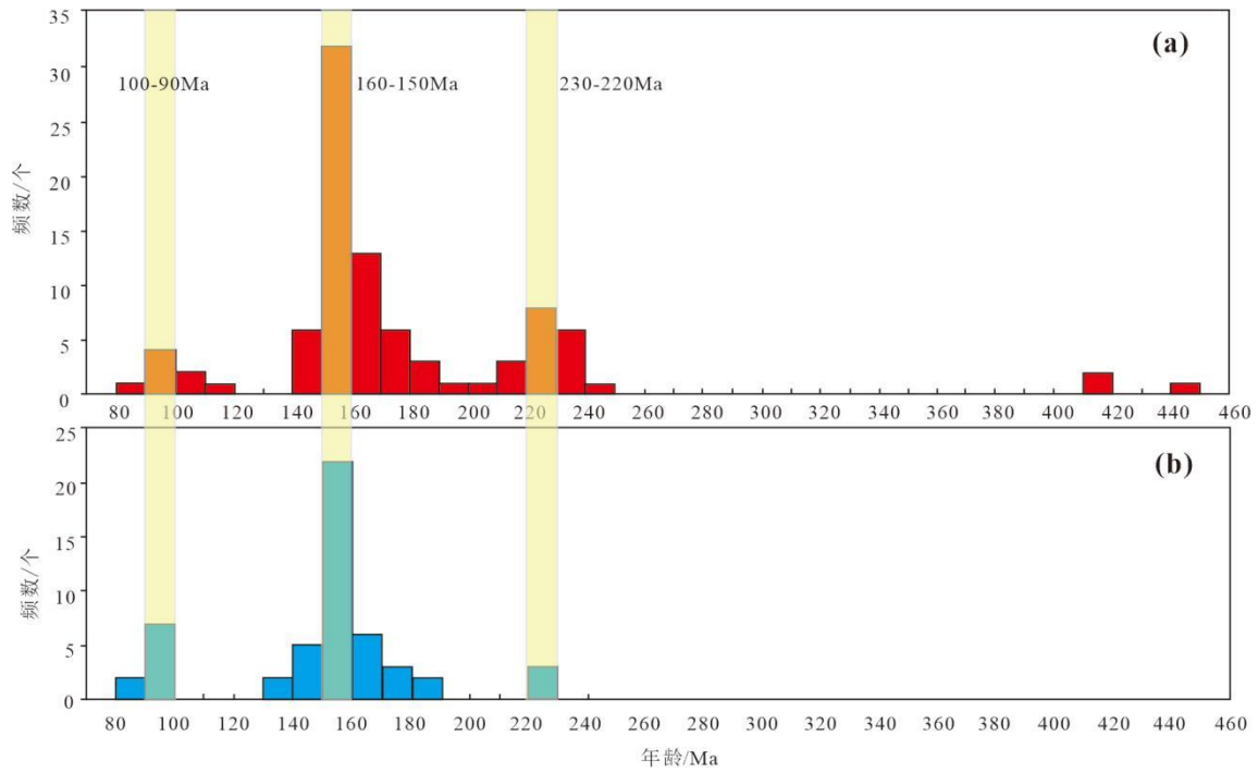
图7 南岭成矿带中段成岩、成矿年龄直方图 (a) 成岩时代; (b) 成矿时代
