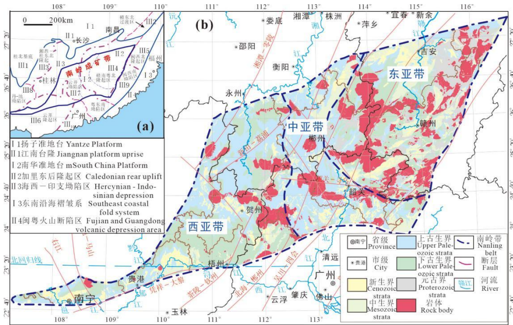
图 1a 南岭成矿带区域构造概略图 (据陈毓川等, 1989; 徐志刚等, 2008); 1b 南岭成矿带地质图 (断裂据黄崇轲等, 1997)
