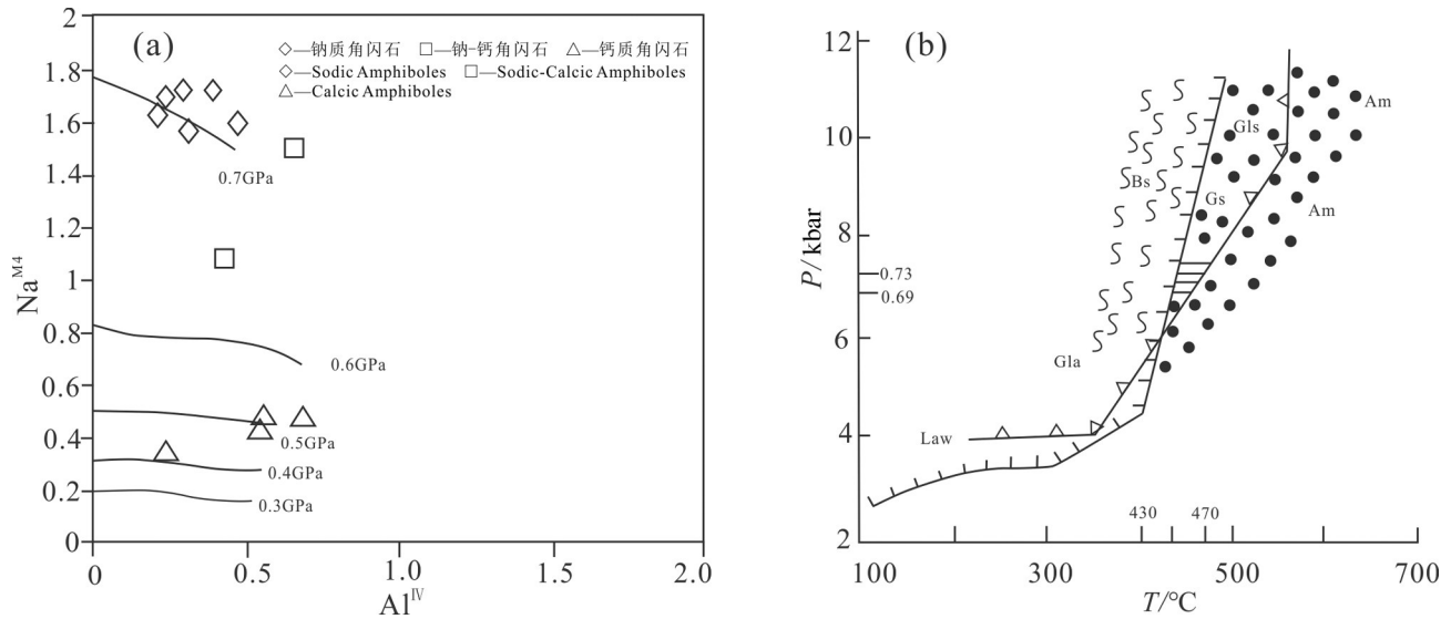
图8 景洪大勐龙地区绿泥绿帘阳起蓝闪片岩角闪石 \text{NaM4}-\text{Al}^{\text{IV}} 相图(a,底图据Brown,1977)蓝闪石变质作用的 P-T 图解(b,底图据Moody et al., 1983)
