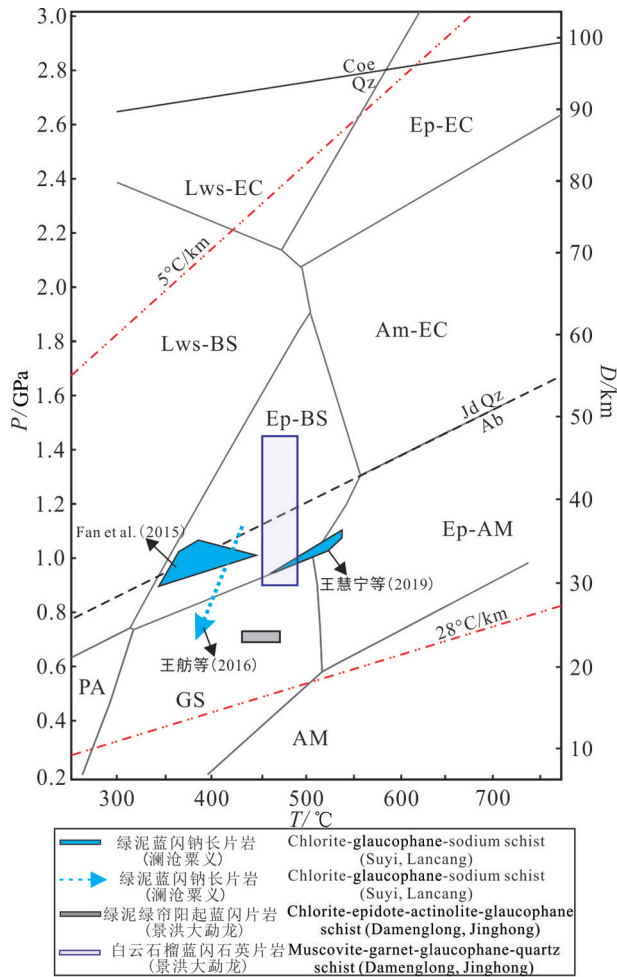
图9 景洪大勐龙地区蓝片岩变质P-T条件估算 变质相系参考Evans(1990)和Liou and Zhang (2003); 变质反 应Coe=Qtz参考Oh and Liou(1998)
