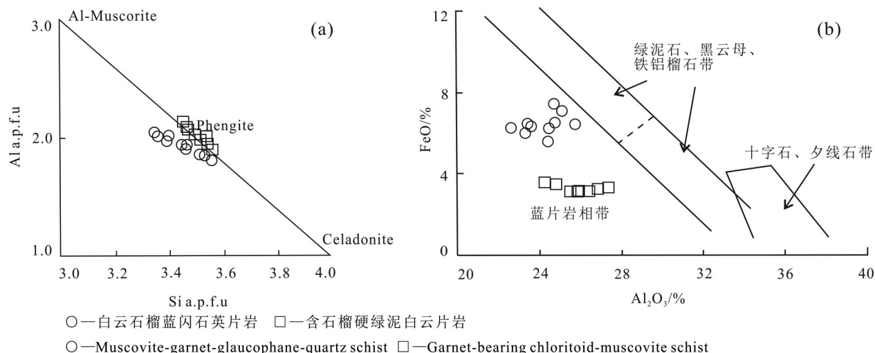
图6 景洪大勐龙勐宋坝地区白云石榴蓝闪石英片岩和含石榴硬绿泥白云母片岩中白云母Al-Si图解(a, 魏春景和朱文萍, 2007)和Al 2 O 3 -FeO图解(b, Miyashiro, 1979)
