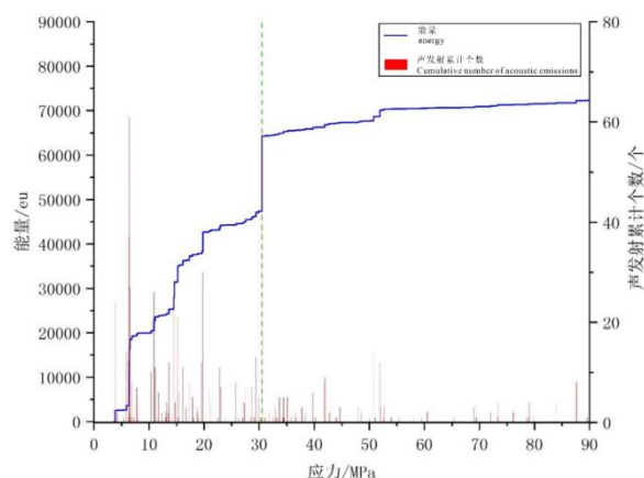
图 3DB13 井太 2 段 2 号样品 45° 声发射曲线图
