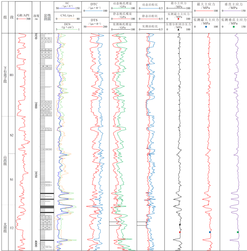
图 4DB23 井上古生界单井地应力剖面
