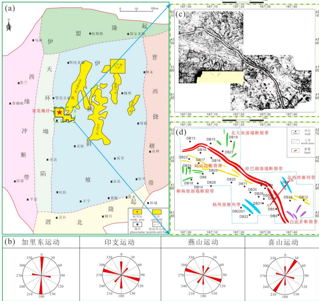
图 1 研究区地质背景图
