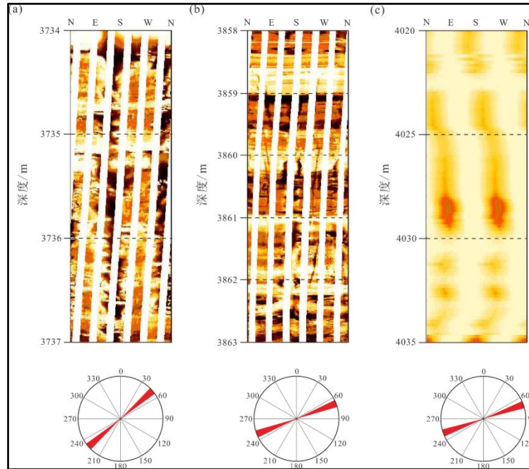
图 5 地应力方向测井解释结果图
