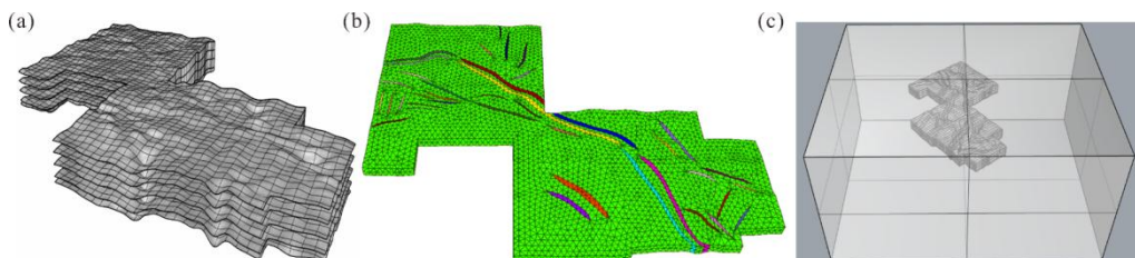
图 7 研究区地质模型图
