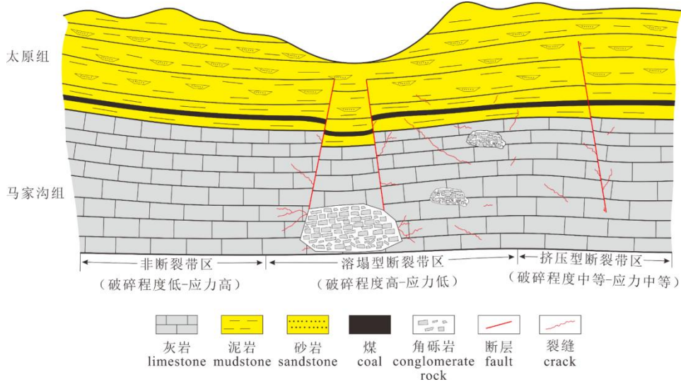
图 10 不同成因断裂带应力扰动模式图
