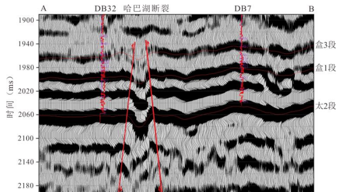
图 2 研究区哈巴湖断裂典型剖面 (剖面位置见图 1d)
