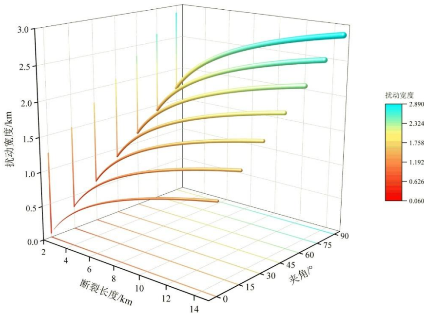
图 14 扰动宽度三维计算图版
