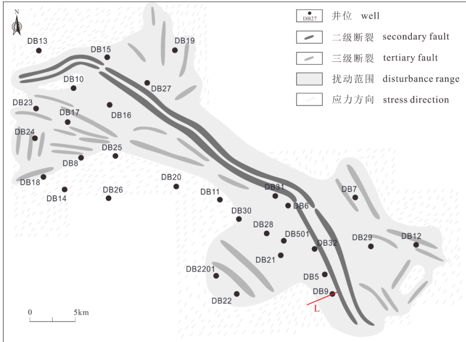
图 12 定北地区地应力扰动带平面分布图
