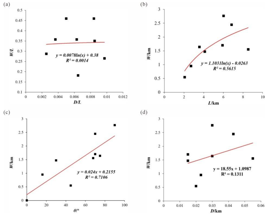
图 13 扰动宽度影响因素分析
