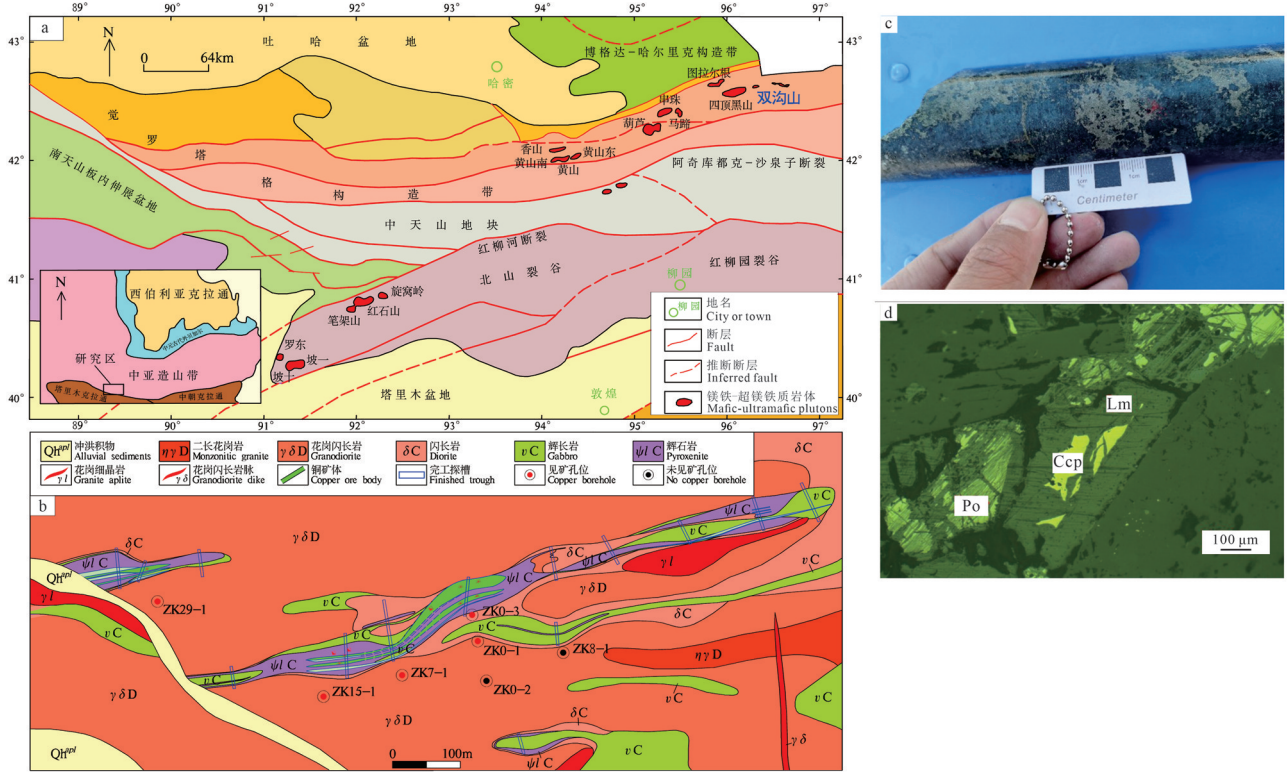
图1 双沟山铜镍矿地质简图及矿石特征
