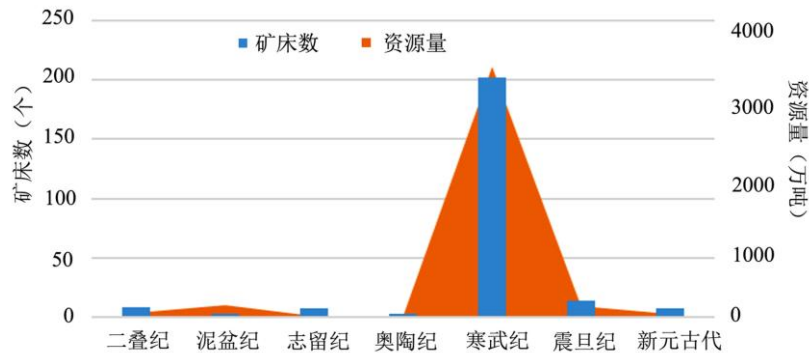
图 4 沉积型钒矿床的成矿时代及对应的资源量
