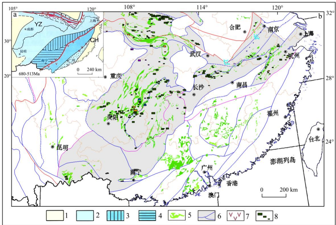
图 8 华南寒武系地层与沉积型钒矿分布图
