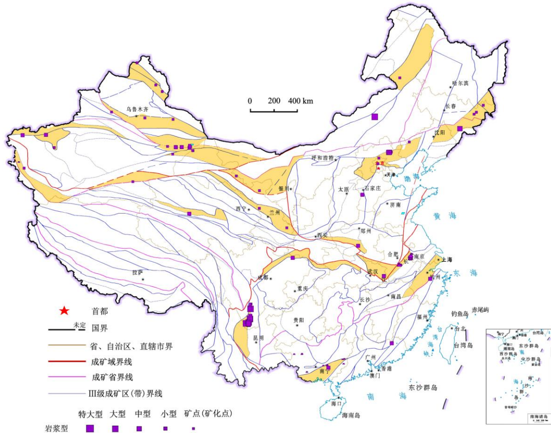
图 6 岩浆型钒矿分布范围
