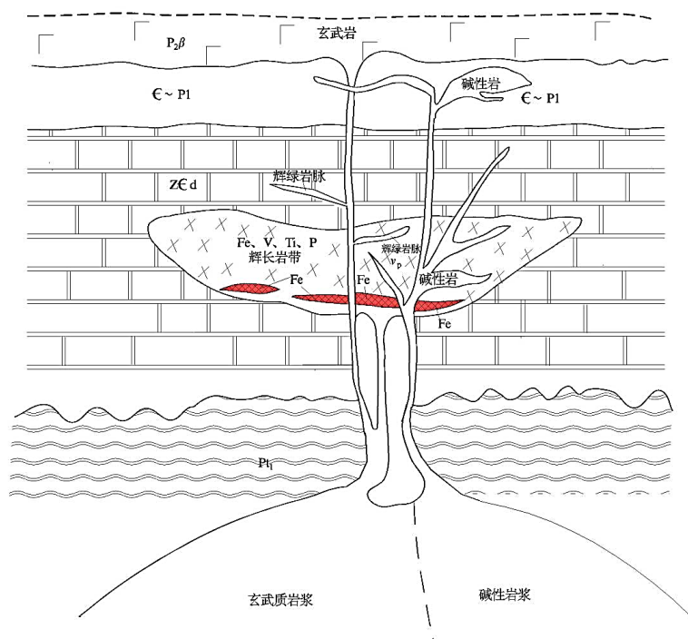
图 10 攀枝花矿床成矿模式图（据四川省潜力评价成果报告） Fig.10 Metallogenic model of Panzhihua magmatic Fe-V-Ti deposits
