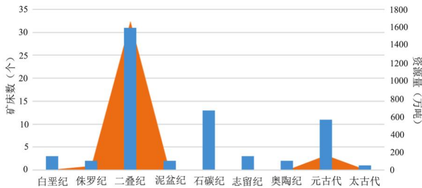
图7 岩浆型钒矿床的成矿时代及对应的资源量
