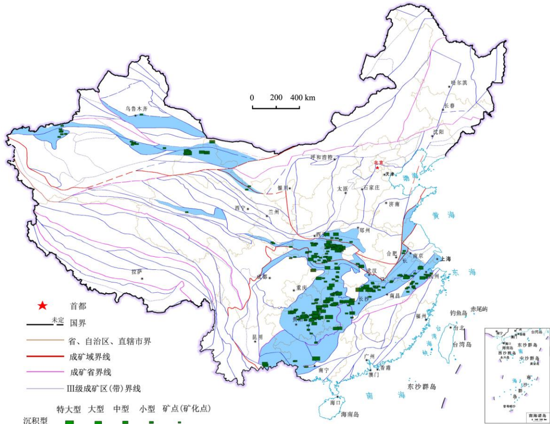
图 3 沉积型钒矿分布范围
