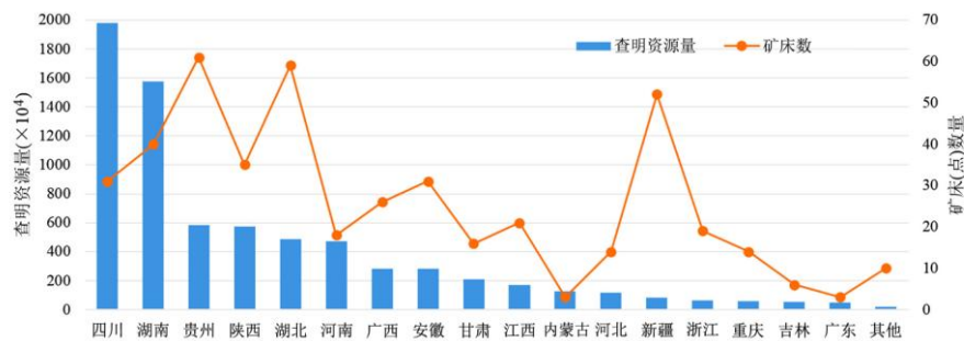
图 1 中国钒矿查明资源分省分布图
