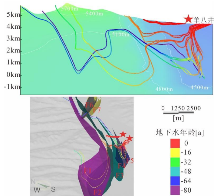
图6 羊八井热泉剖面地下水流线和地下水流动三维路径
