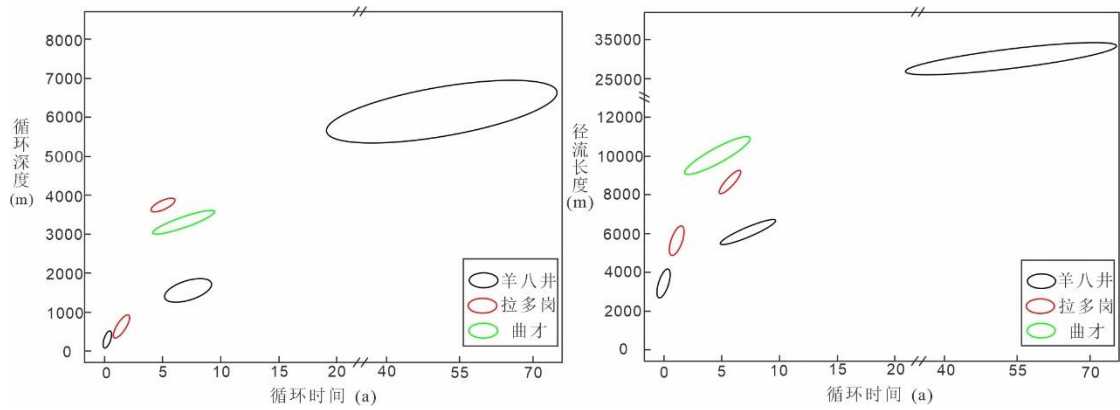
图9 三个热泉地下水模拟结果汇总
