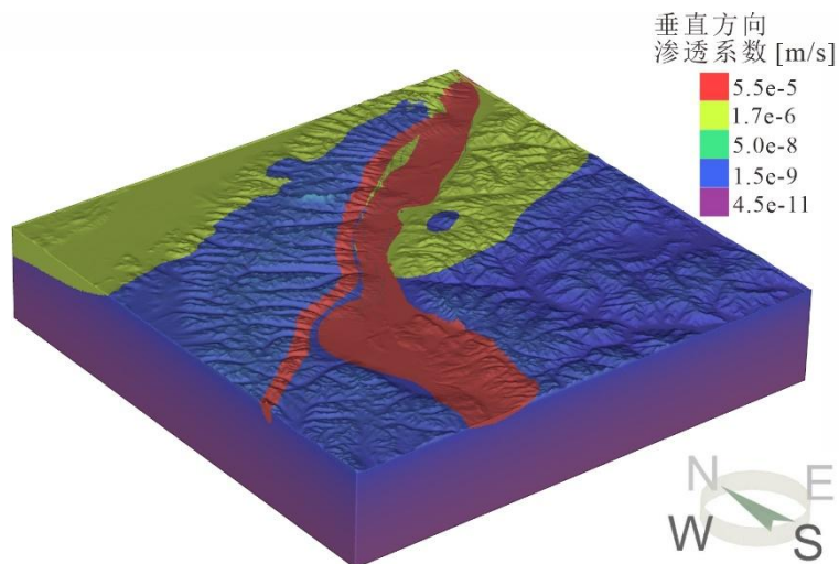
图 4 模型垂直渗透系数
