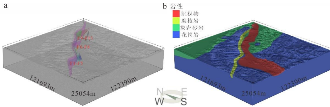
图 2 包括断层（彩色）的三维地质简化模型（a）和模型岩性单元设置（b）
