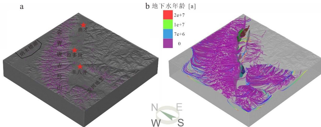
图 10 补给高程高于 5500m 区域位置 (a) 和补给高程高于 5500m 以上的地下水流线模拟结果 (b)
