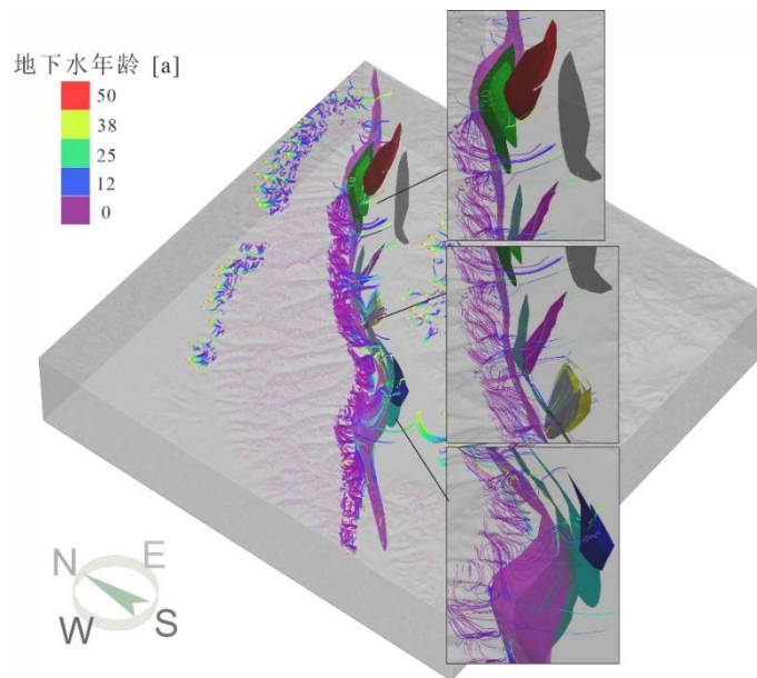
图 12 补给高程高于 5500m 的地下水流线 50 年年龄模拟结果
