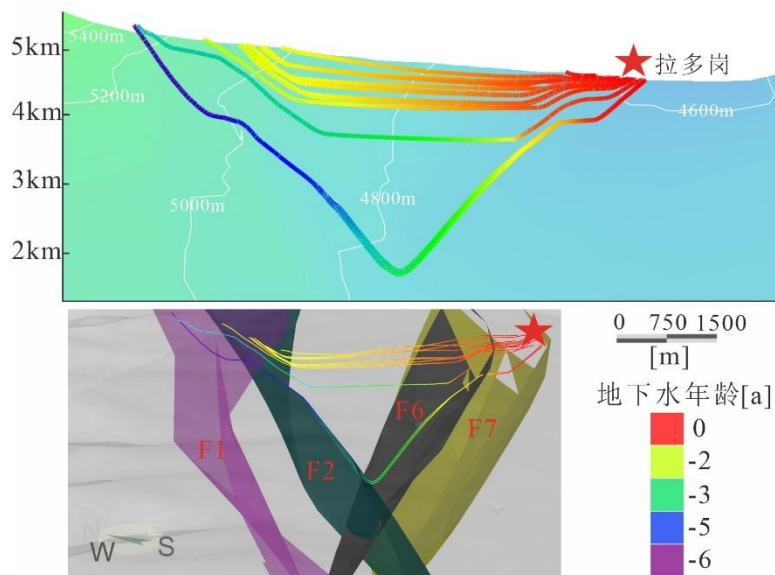
图 7 拉多岗热泉剖面地下水流线和地下水流动三维路径
