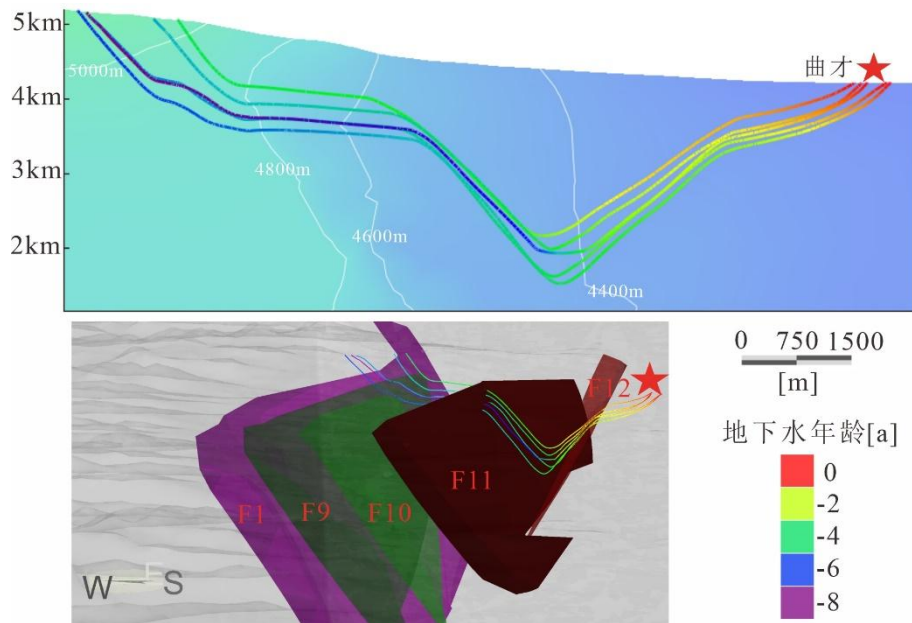
图 8 曲才热泉剖面地下水流线和地下水流动三维路径
