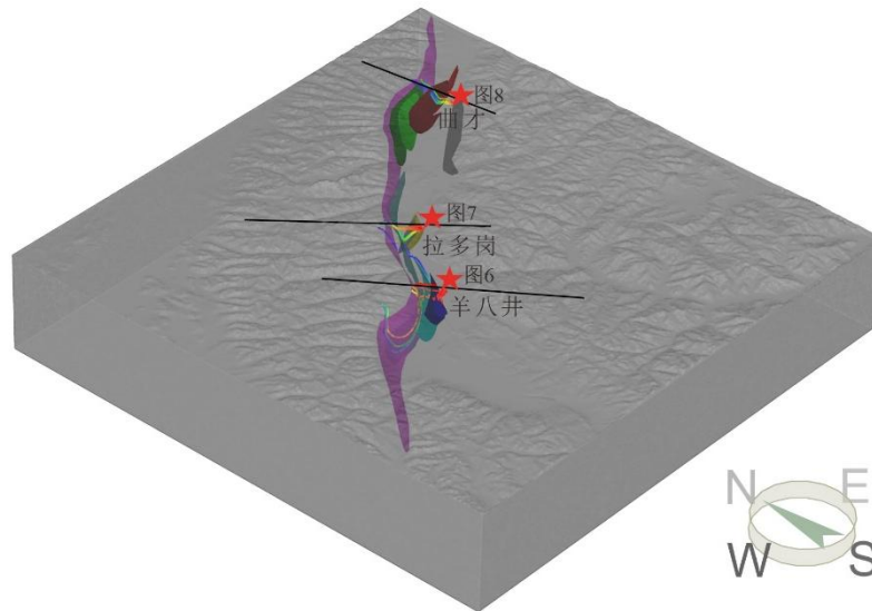
图 5 热泉地下水模拟结果及图 6-8 测线剖面位置
